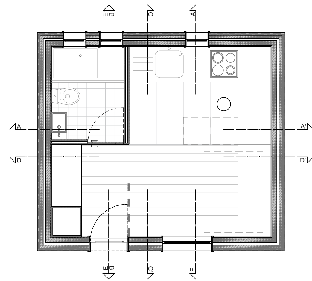
9. Planta tipo A | 1/50
