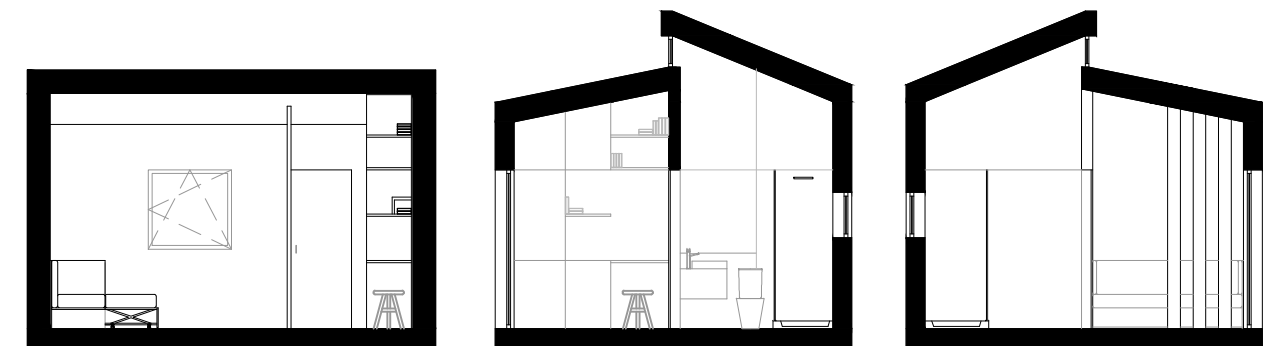
6. Corte DD' | 1/100
