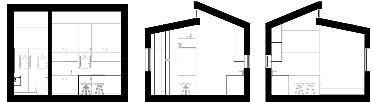
3. Corte AA' | 1/100
