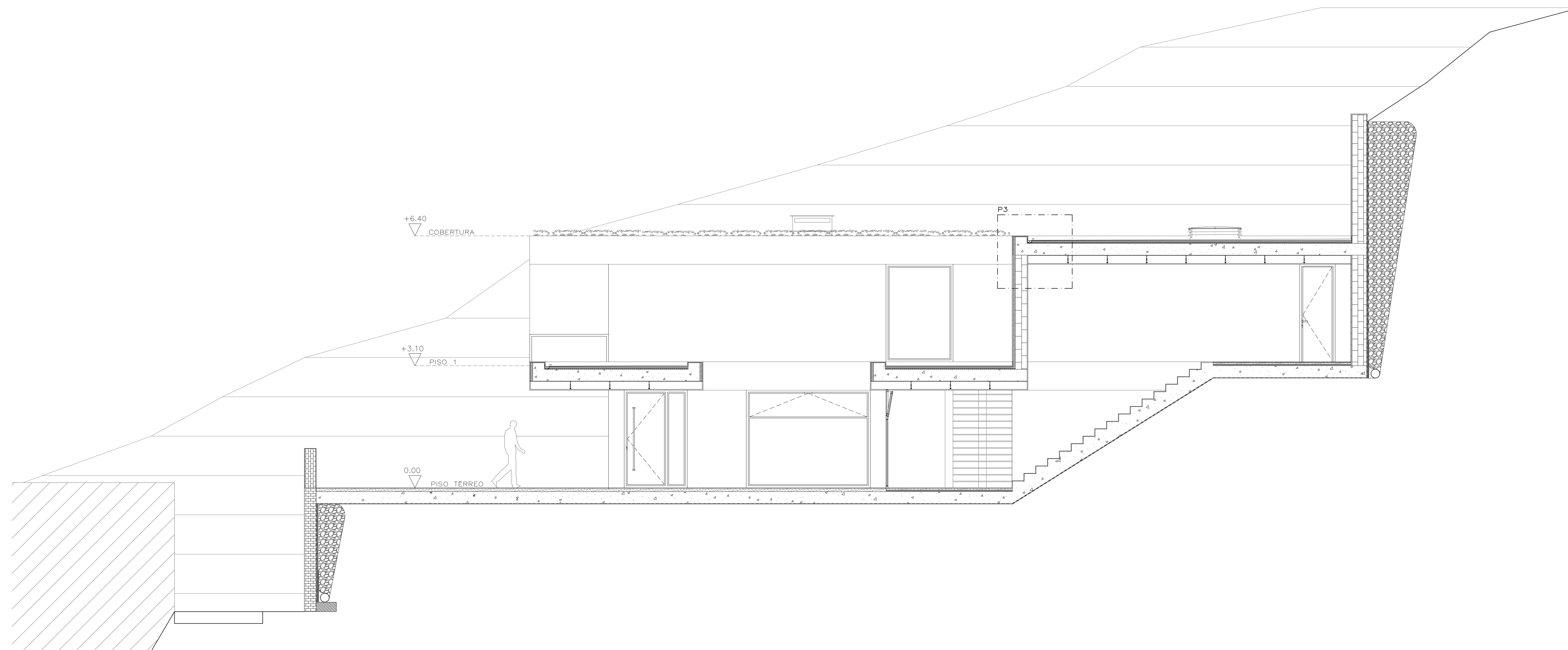
CORTE AA'
