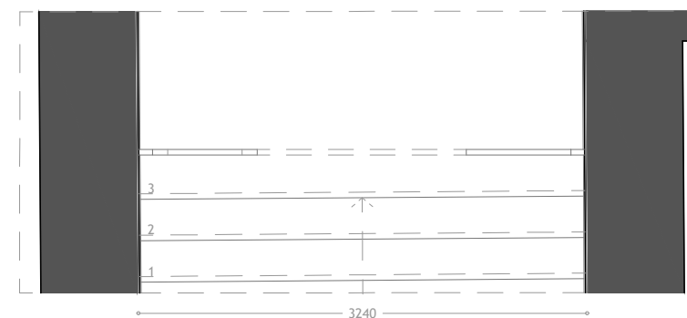
Imagem 160 - Levantamento gráfico da Porta P2 - Planta - Escala 1:50
