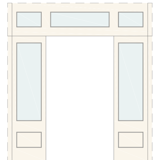
Imagem 162 - Levantamento gráfico a cores da Porta P2 - Traseiras - Escala 1:50
