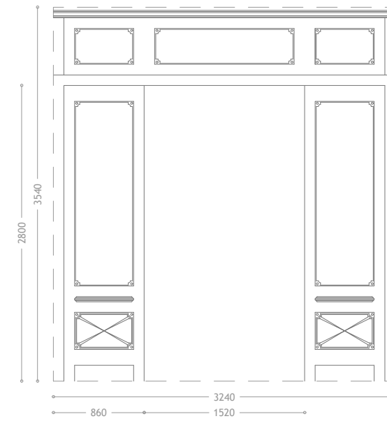
Imagem 158 - Levantamento gráfico da Porta P2 - Frente - Escala 1:50
