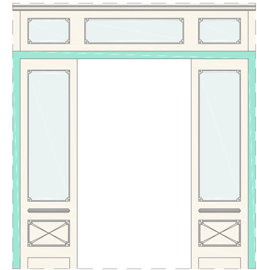
Imagem 161 - Levantamento gráfico a cores da Porta P2 - Frente - Escala 1:50
