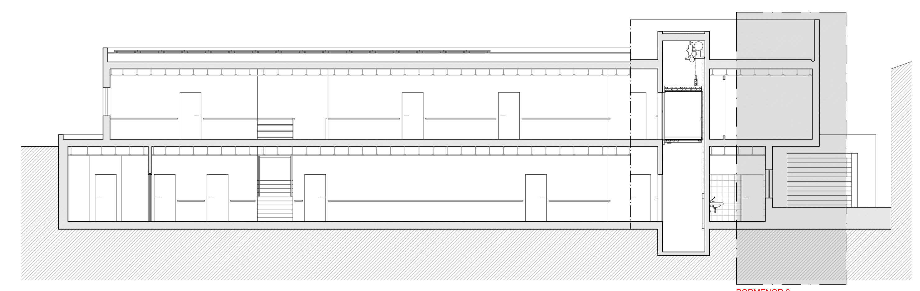
CORTE F-F PROPOSTO
