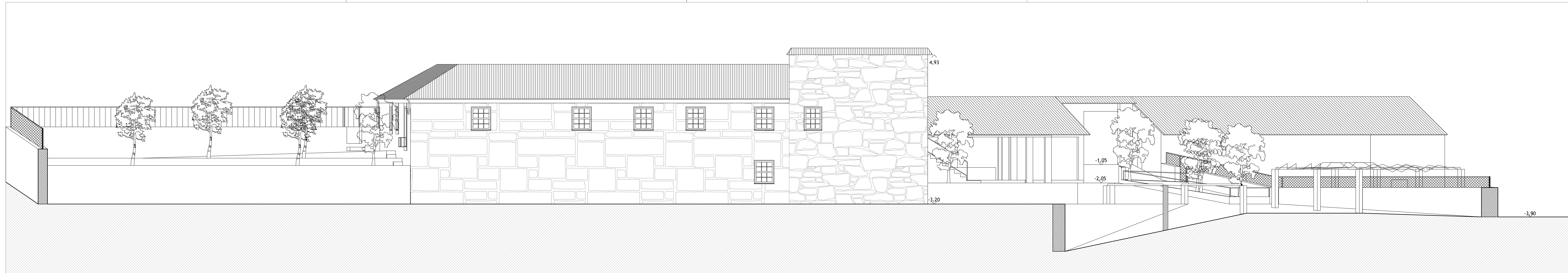
Alçado Principal
