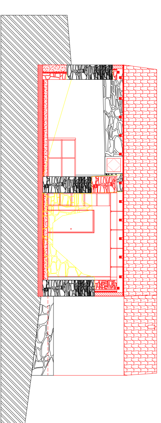
CORTE AA' DE SOBREPOSIÇÃO
