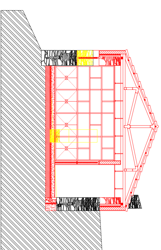
CORTE BB' DE SOBREPOSIÇÃO
