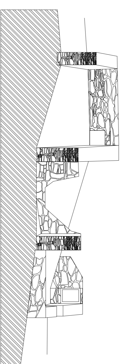
CORTE AA' EXISTENTE
