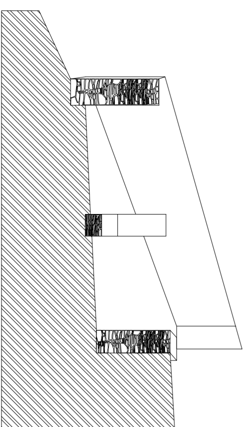
CORTE BB' EXISTENTE
