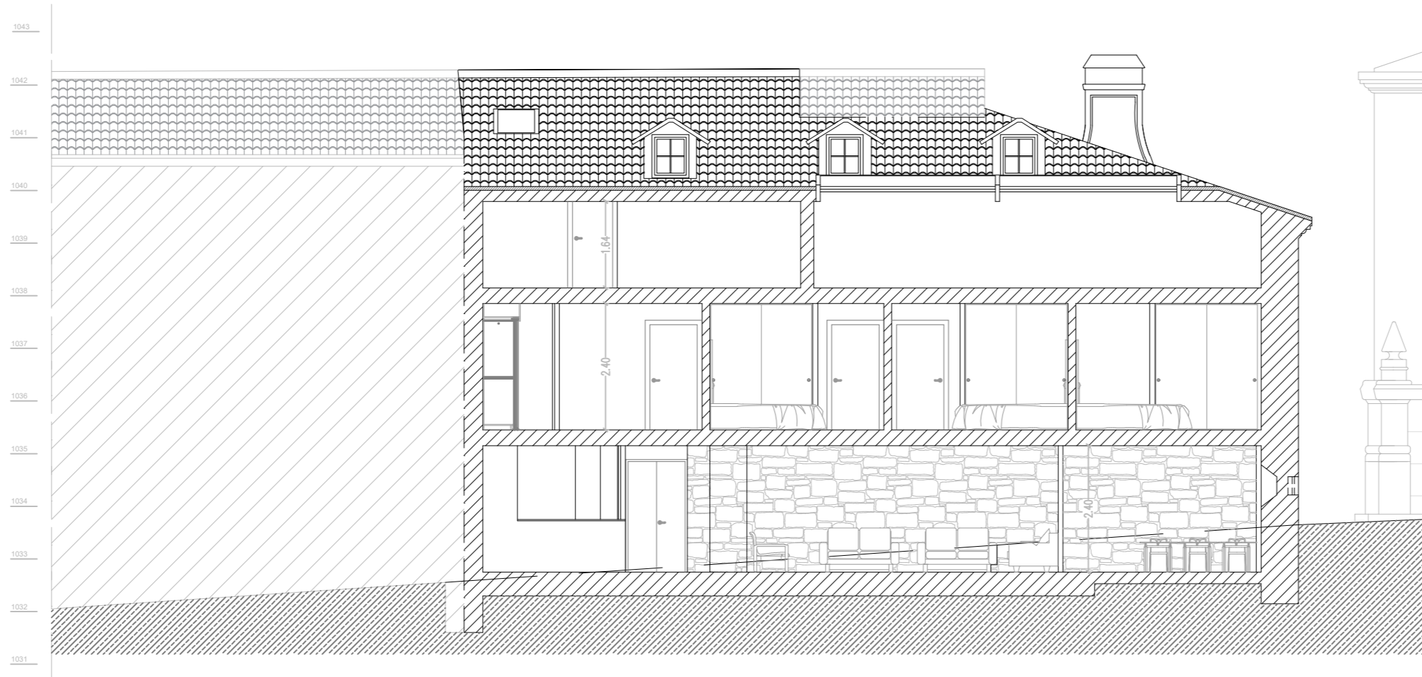
Corte E-F
