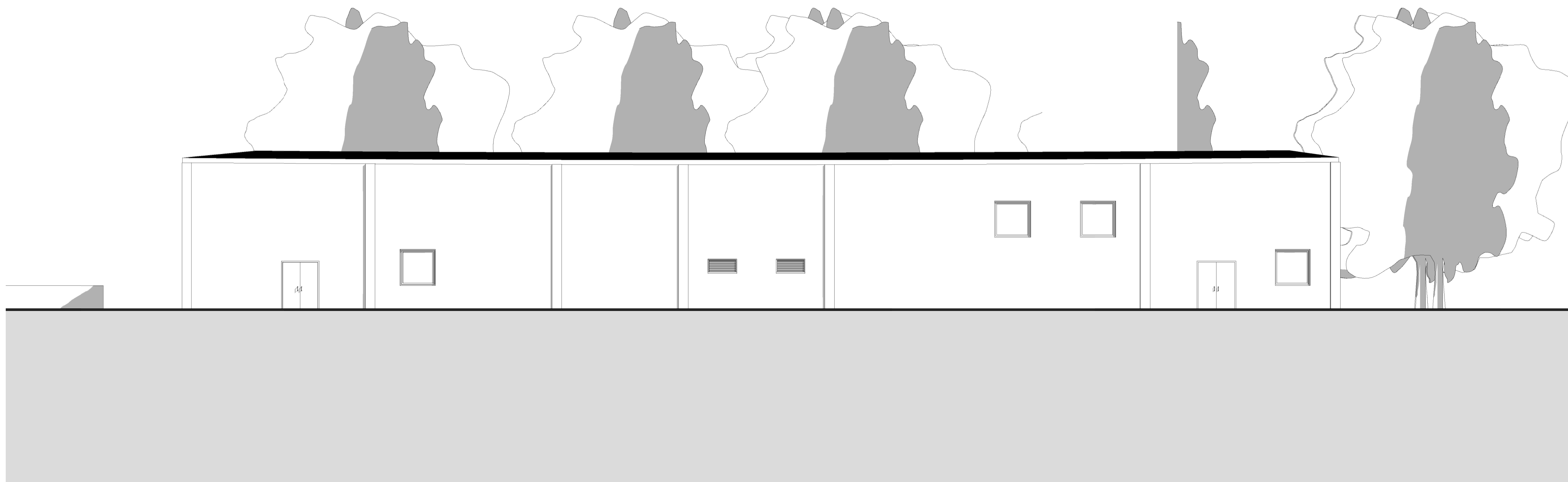
Alçado Oeste
