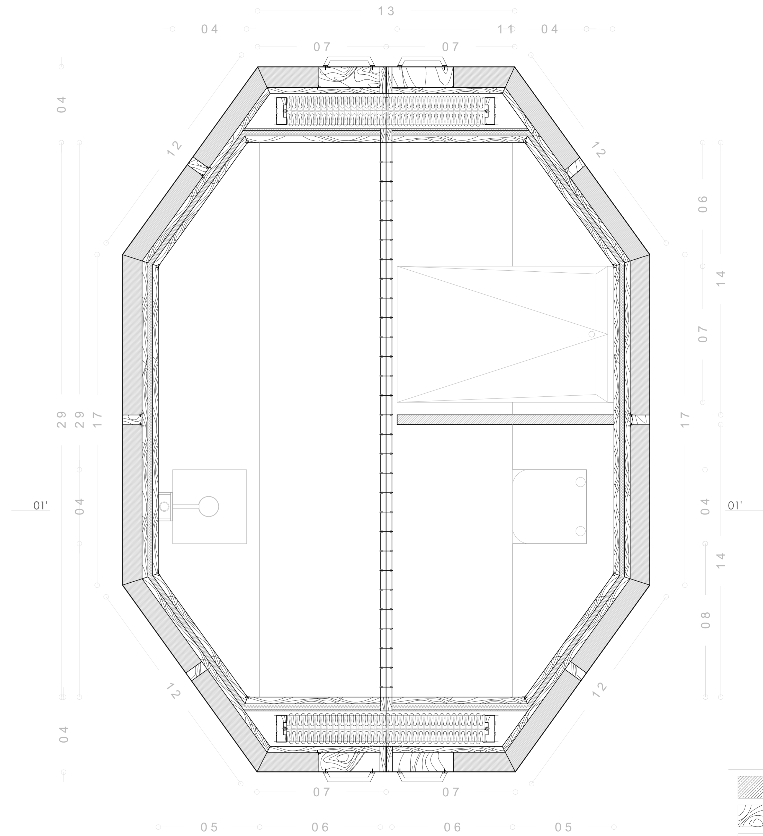
PLANTA 01'
