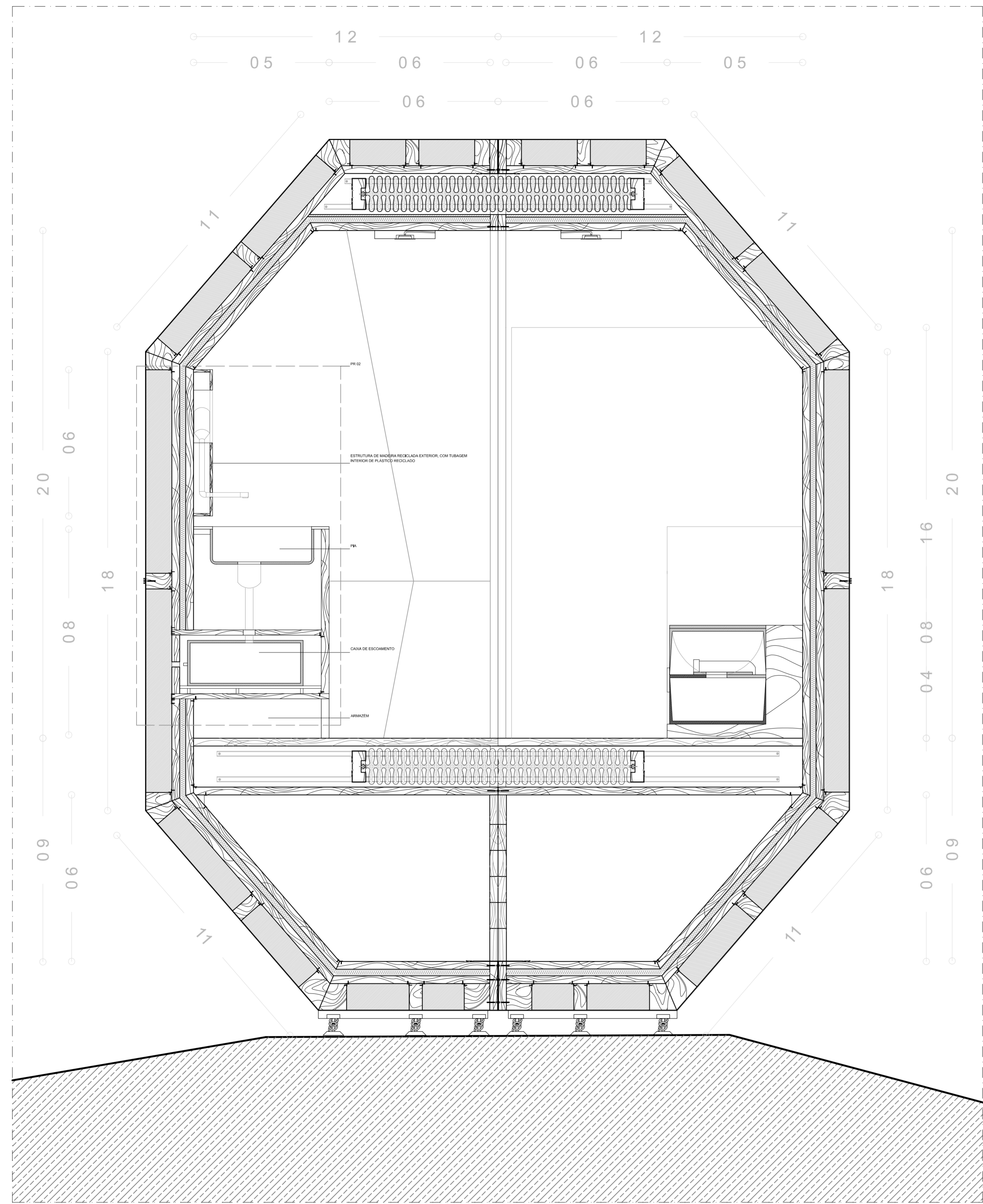
CORTE 1'
