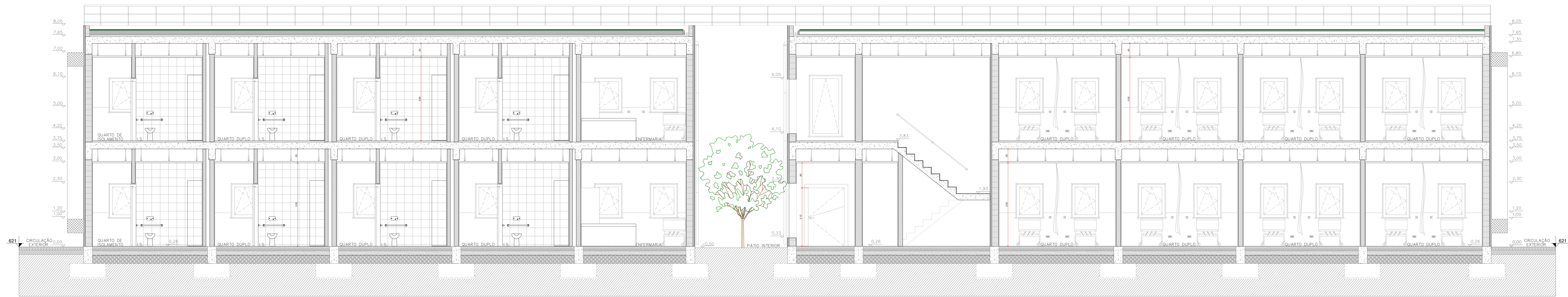
CORTE B.B. 621
