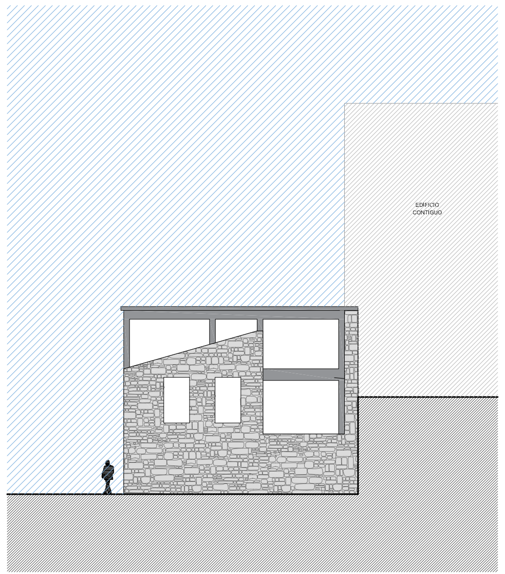
ALÇADO DIREITO
