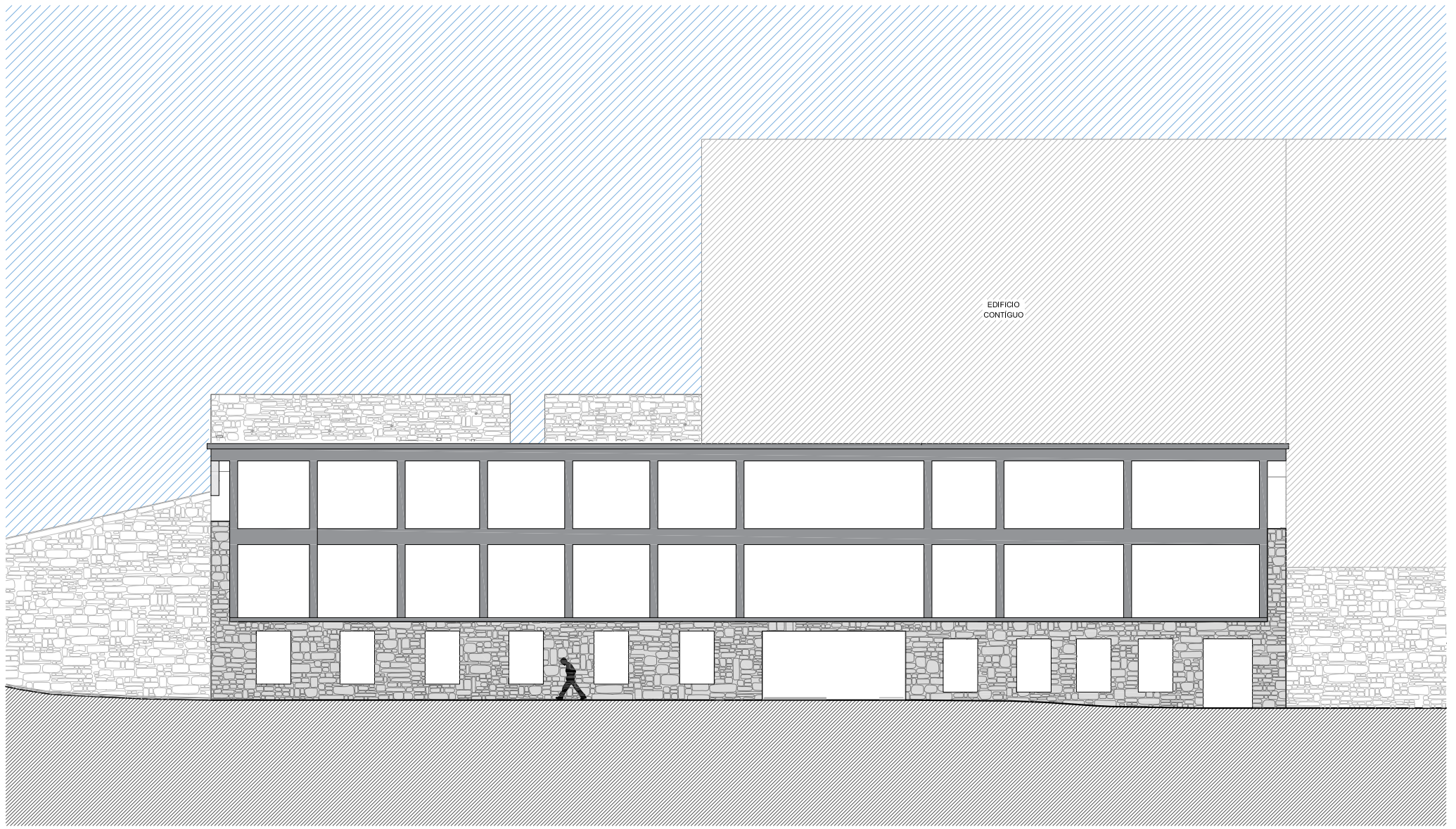
ALÇADO FRONTAL
