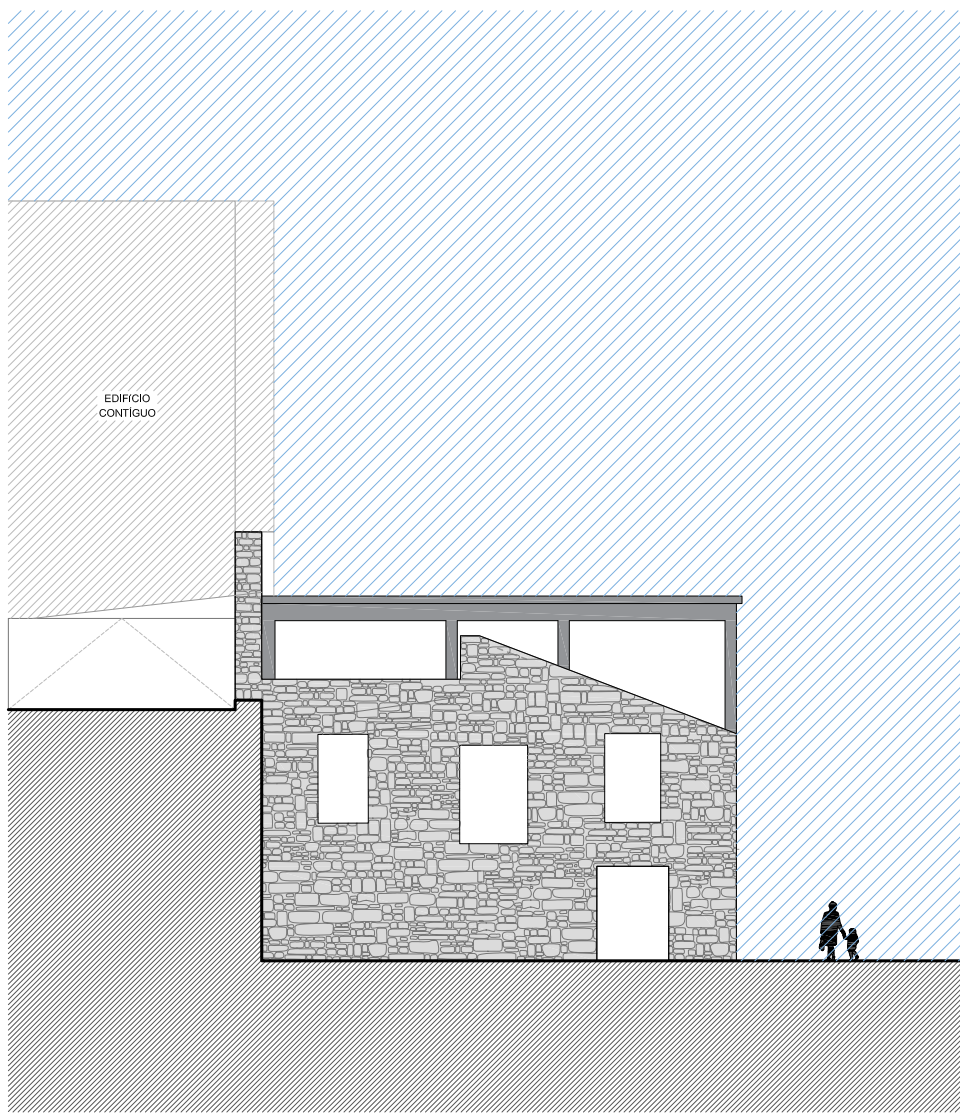
ALÇADO ESQUERDO
