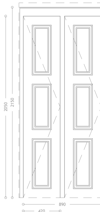
Imagem 254 - Levantamento gráfico da Porta P9 - Frente - Escala 1:25
