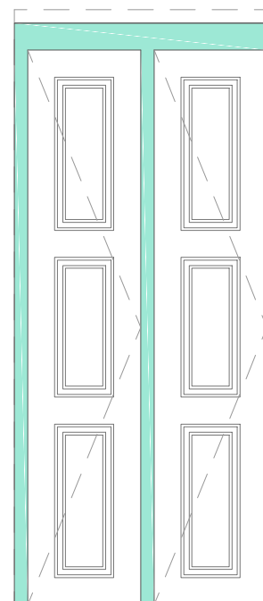
Imagem 256 - Levantamento gráfico a cores da Porta P9 - Frente - Escala 1:25
