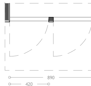
Imagem 255 - Levantamento gráfico da Porta P9 - Planta - Escala 1:25
