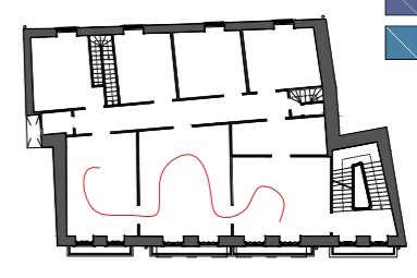
Esquema de Fluxos entre as Salas
