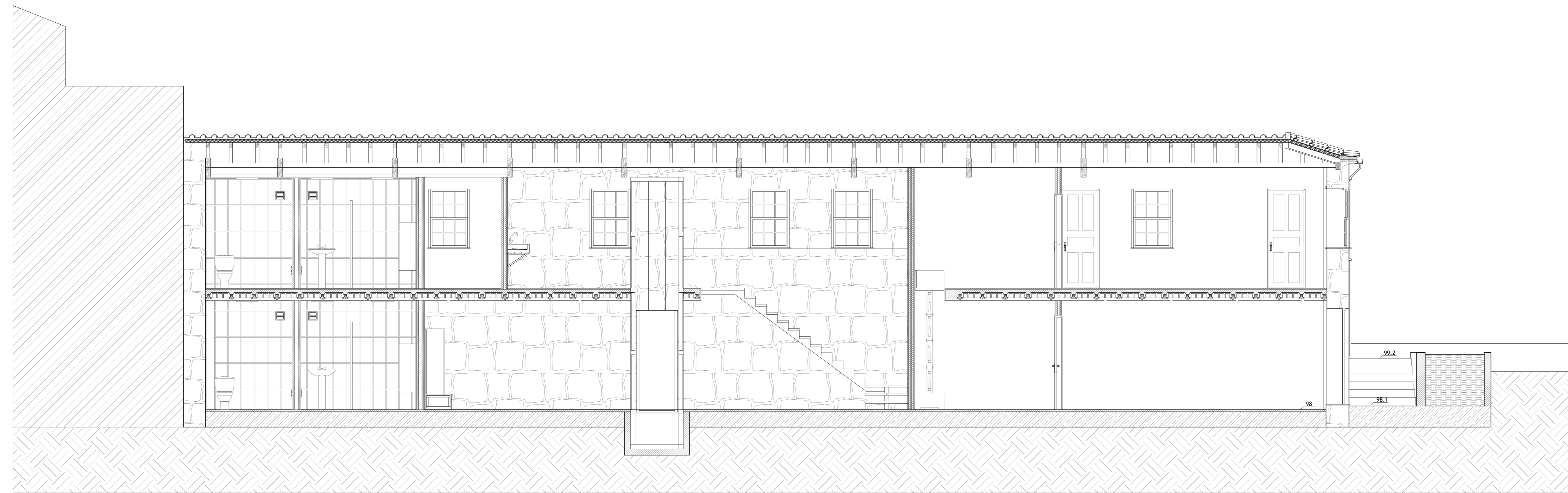
Corte A-A'
