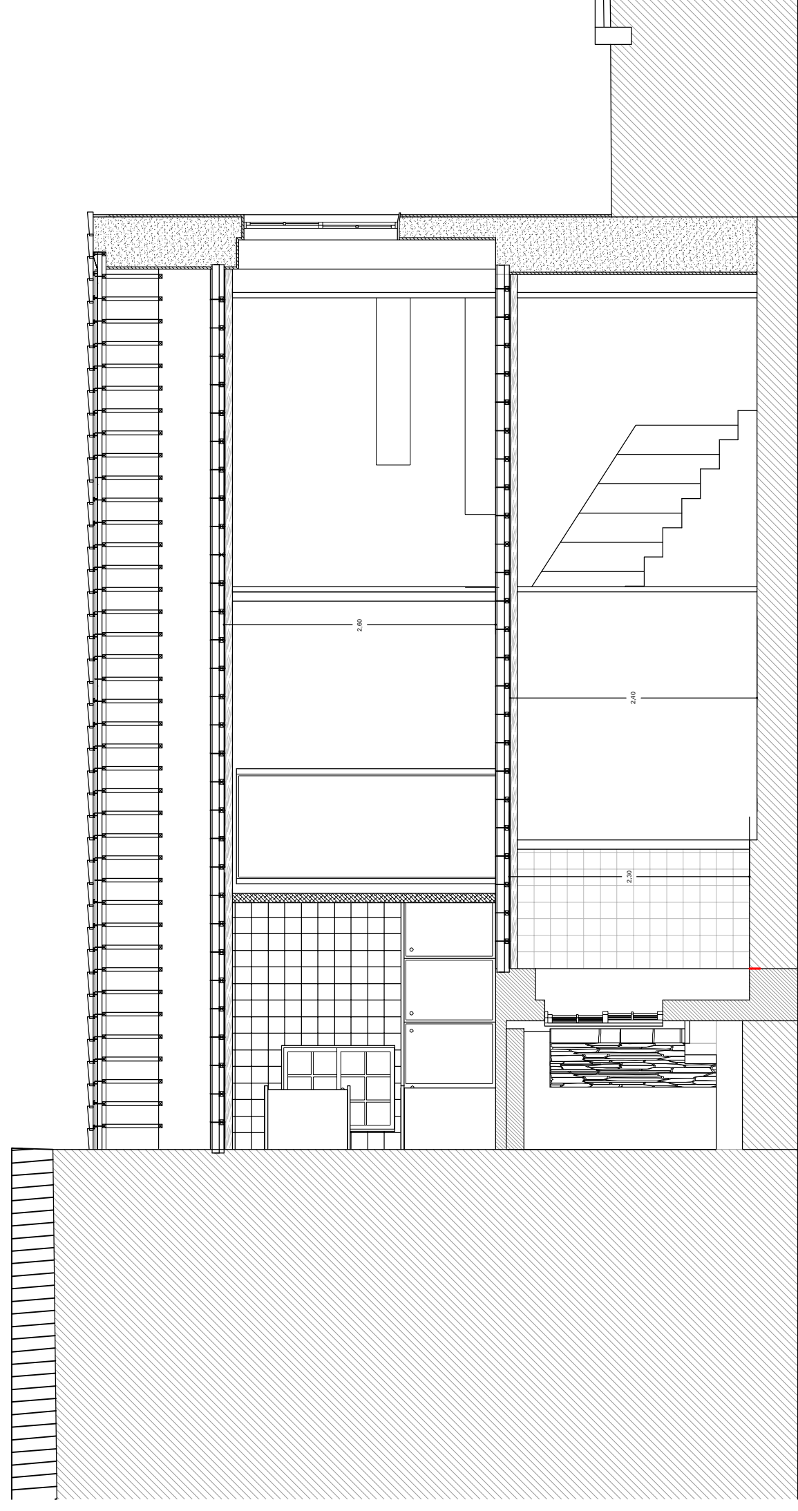
Corte C-C
