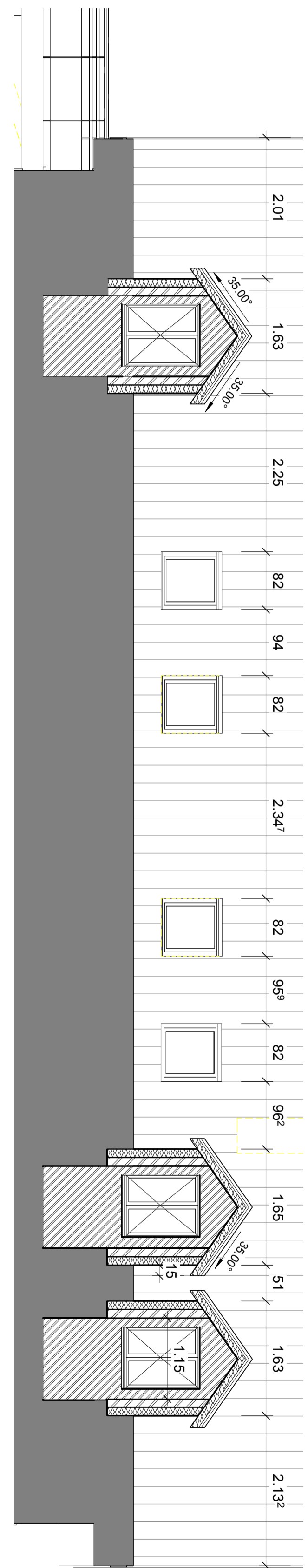
Corte JJ' 1:50
