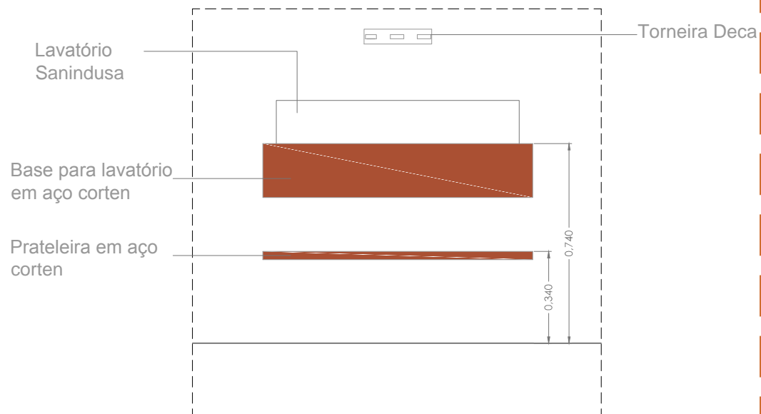
Alçado
