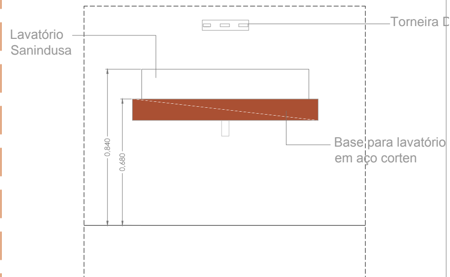
Alçado
