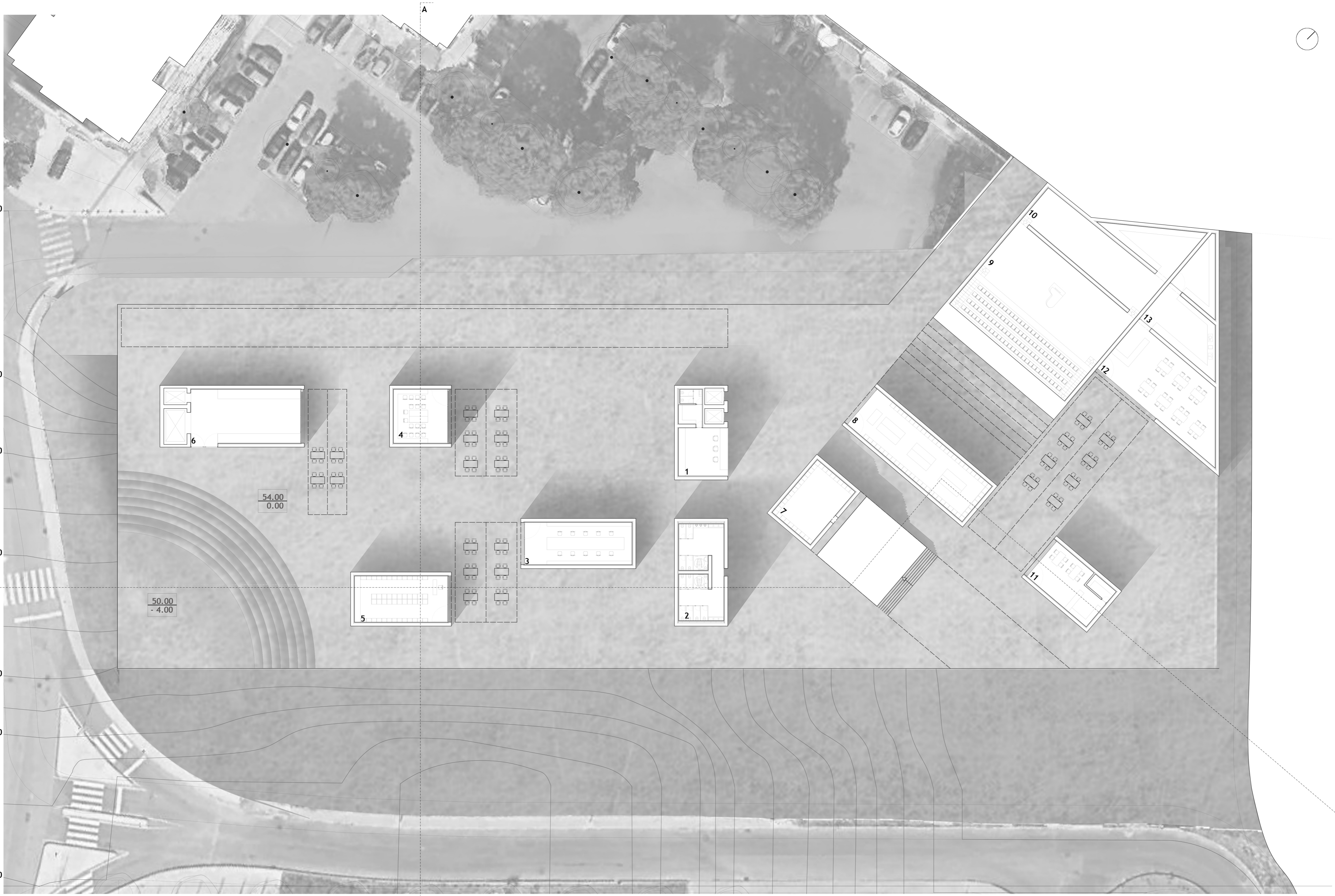
PLANTA PISO 0 ESCALA 1:300 1-QUIOSQUE; 2-SANITÁRIOS; 3-ESPAÇO DE OCUPAÇÃO DE TEMPOS LIVRES; 4-CENTRO DE CONVÍVIO; 5-LIVRARIA; 6-ESPAÇO SERVIDOR DE ANFITEATRO; 7-ARRUMOS; 8-MINIMERCADO; 9-AUDITÓRIO; 10-ESPAÇO SERVIDOR DE AUDITÓRIO; 11-CAFÉ; 12-RESTAURANTE; 13-ESPAÇO SERVIDOR DE RESTAURANTE; 14-FOYER; 15-RECEÇÃO; 16-ESPAÇO DE SERVIÇOS DE SALAS DE AULAS/WORKSHOPS; 17-SALAS DE AULAS/WORKSHOPS; 18-BILHETEIRA/RÉGIE; 19-BILHETEIRA; 20-SALA DE EXPOSIÇÕES; 21-ARQUIVO; 22-ÁREA DE CONVÍVIO
