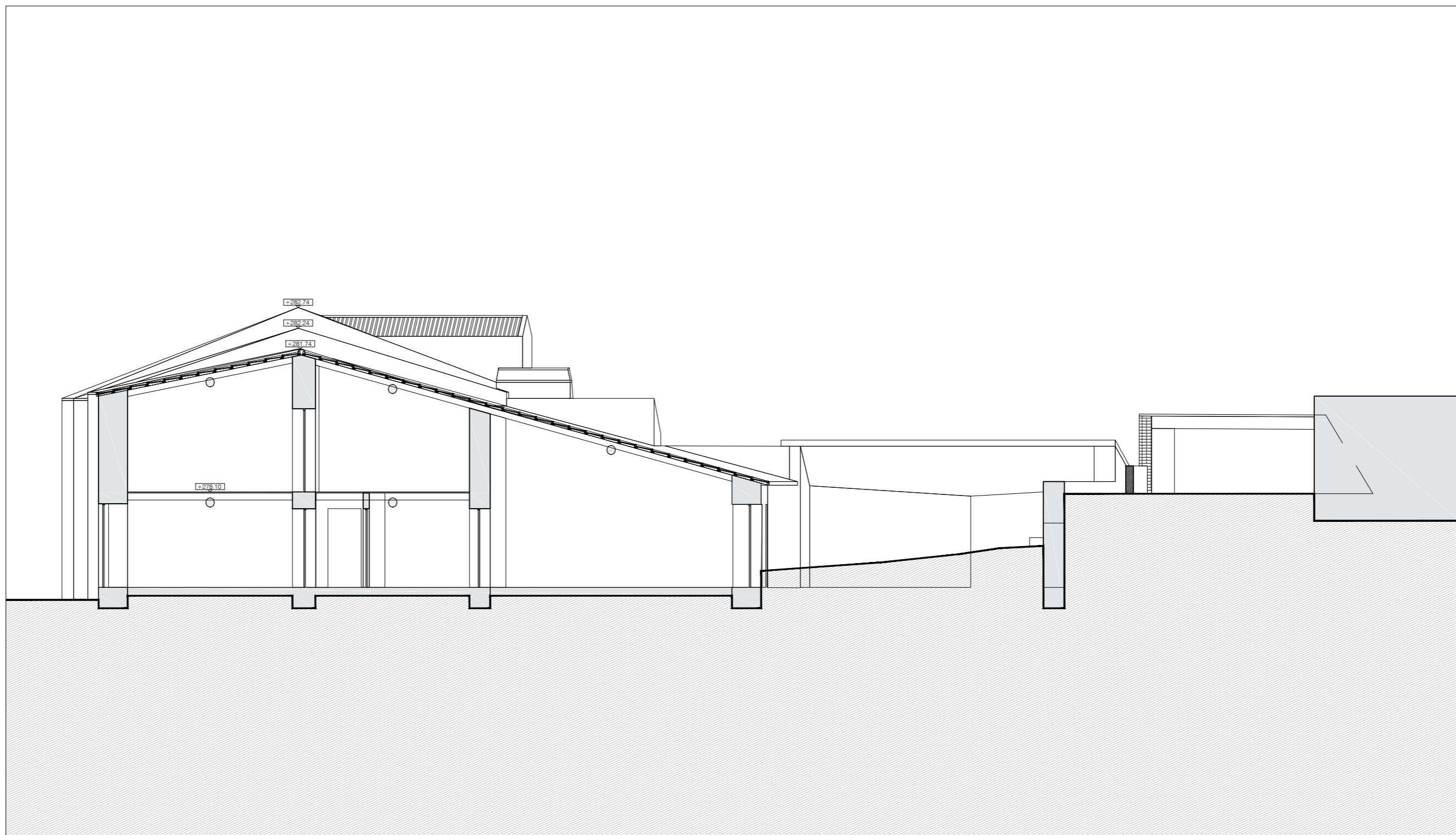
CORTE N1 ANEXO CASA PINA FALCÃO
