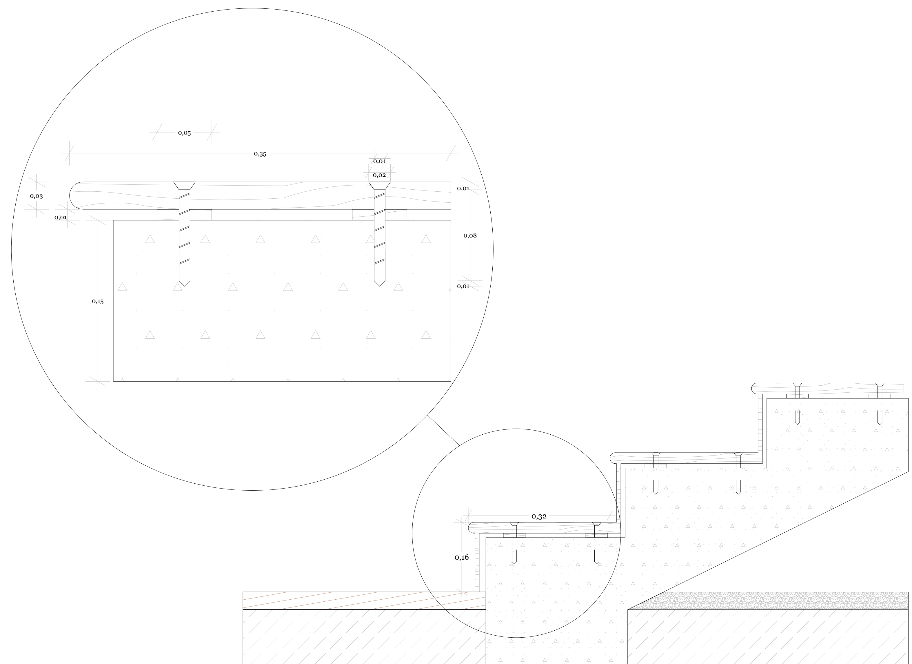
Vista Lateral da Escada - Detalhe 1:5 / 1:2
