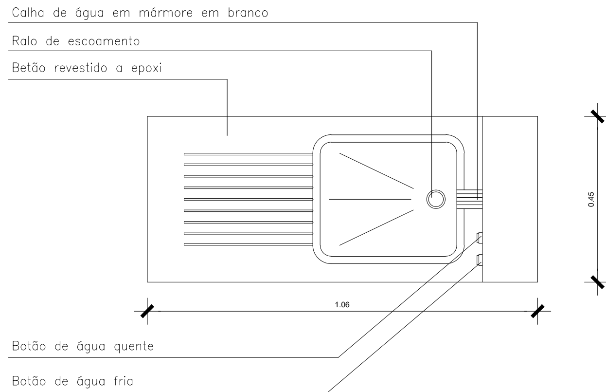
Planta
