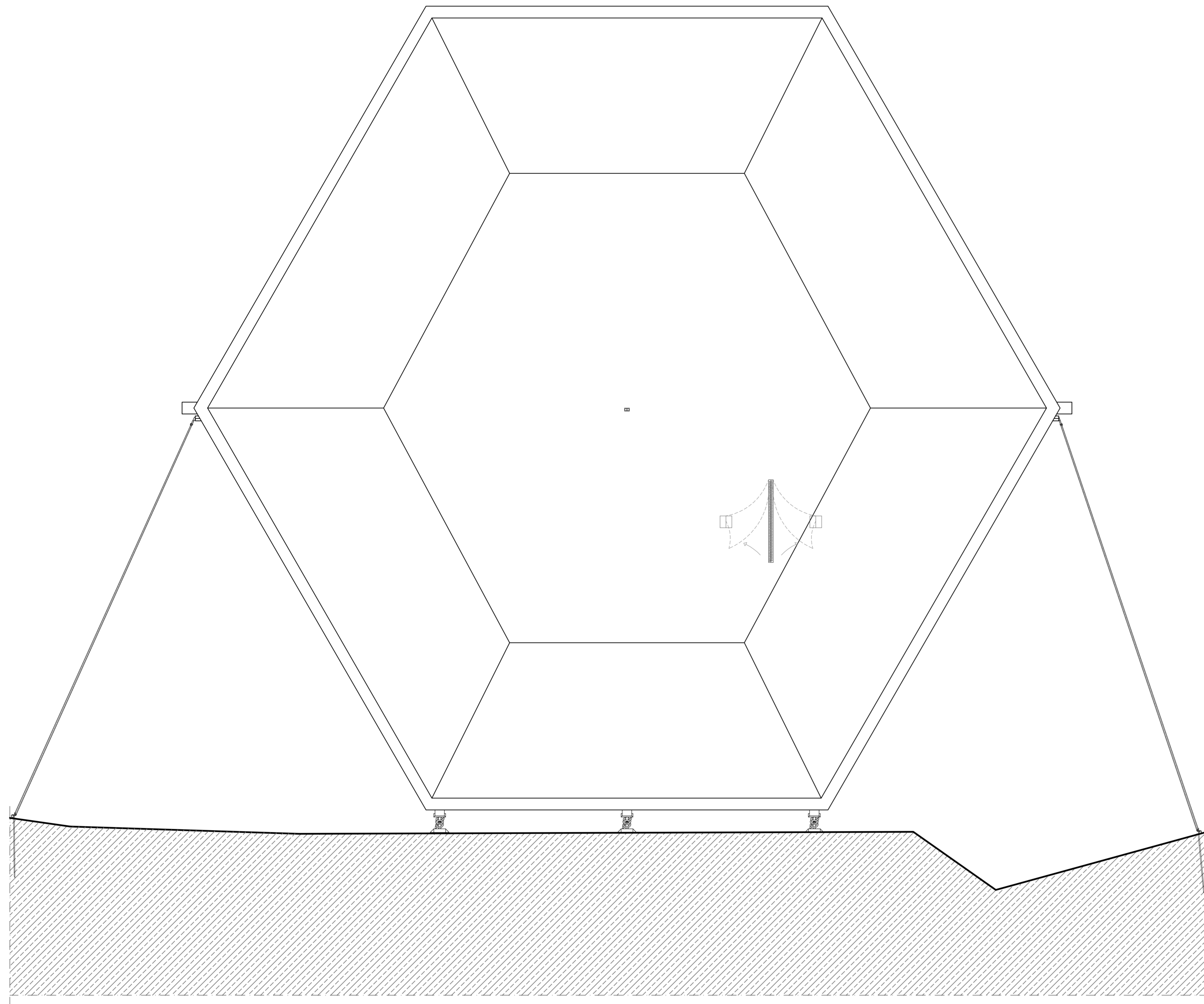
ALÇADO 02
