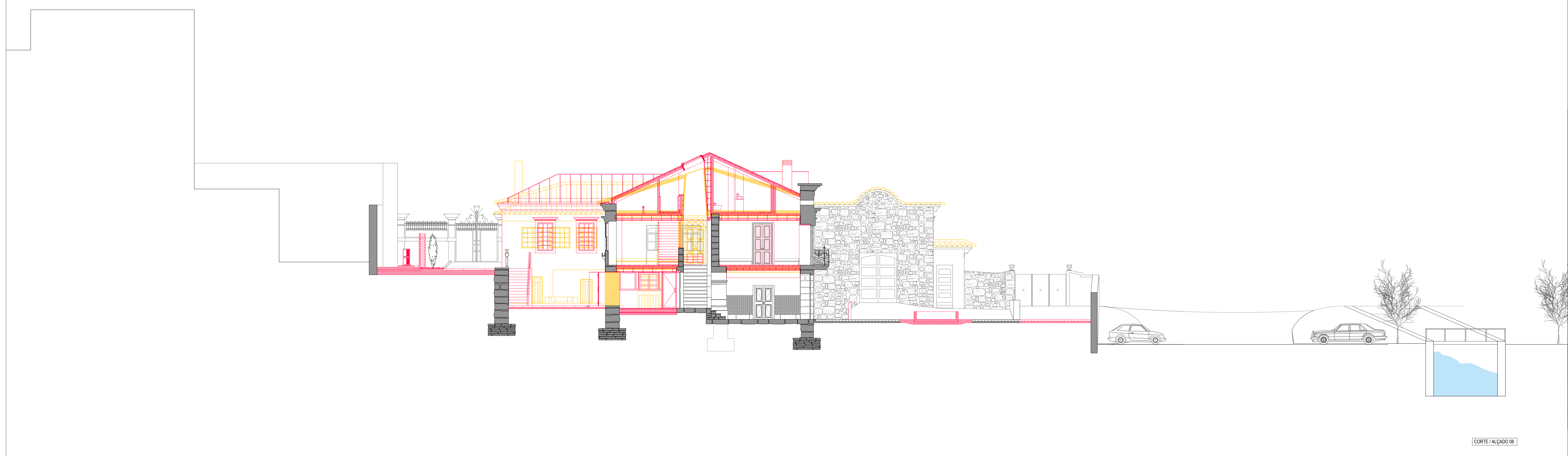
CORTE / ALÇADO 07
