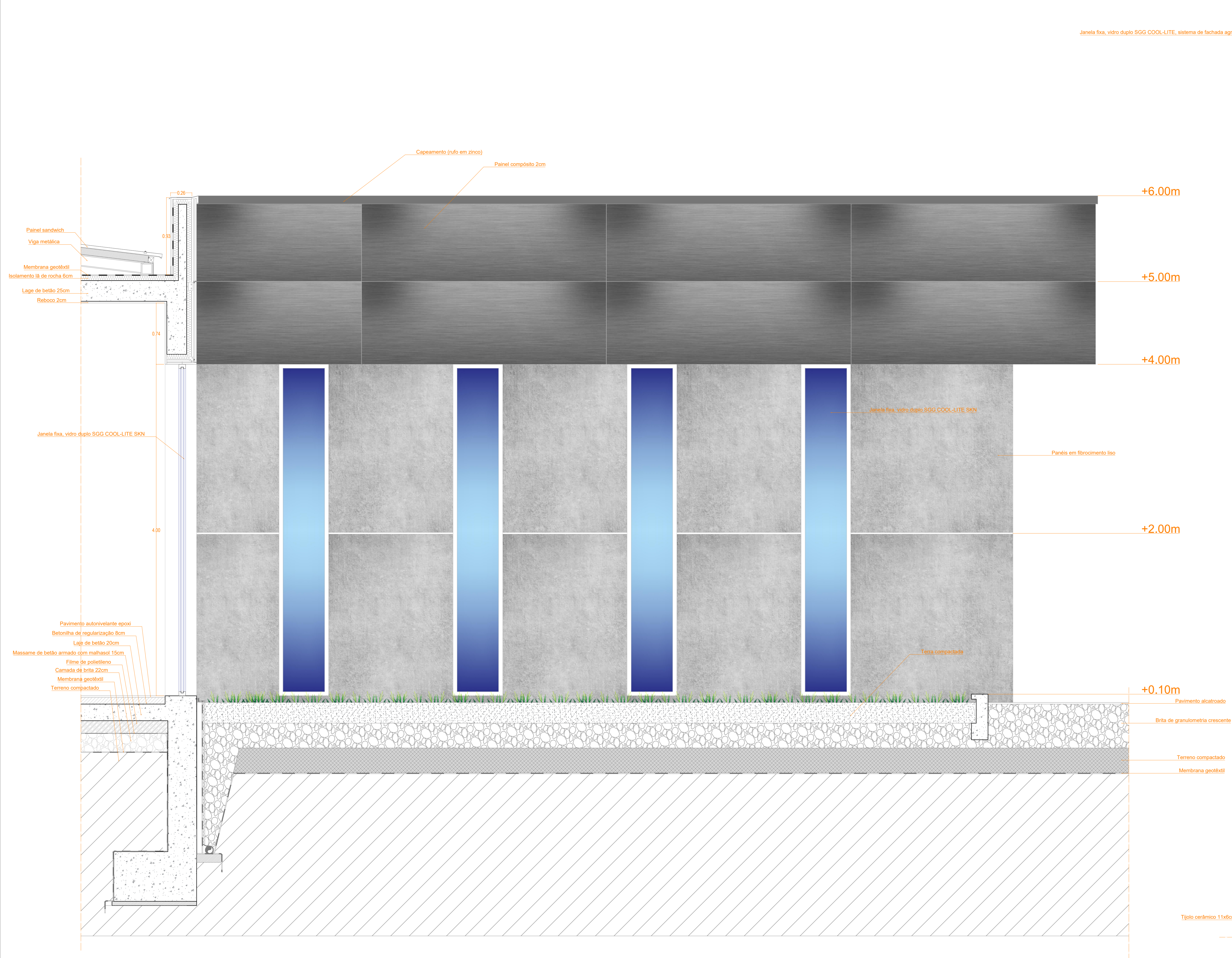
CORTE - A - A' DETALHE ESC.: 1 / 20
