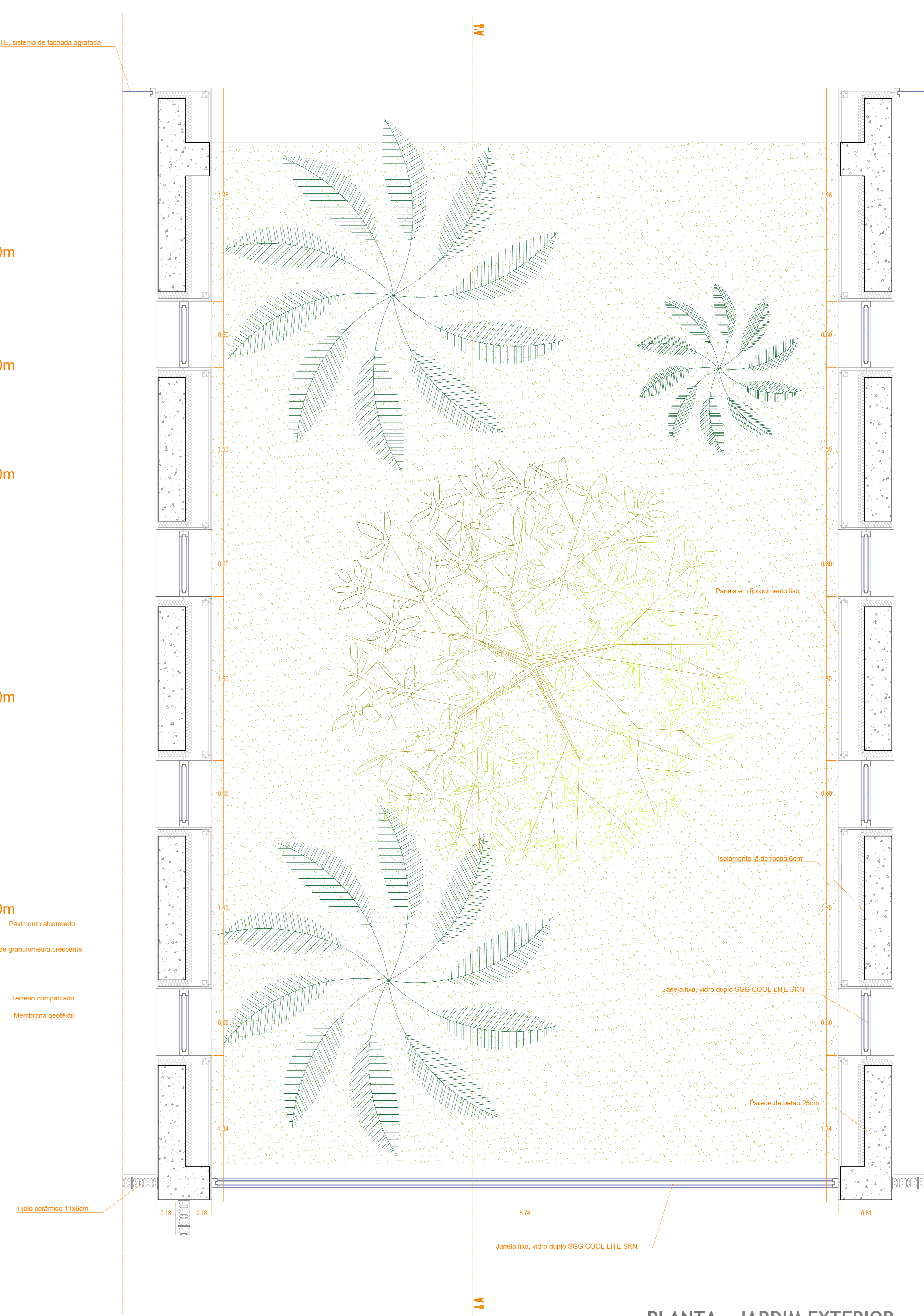
PLANTA - JARDIM EXTERIOR DETALHE ESC.: 1 / 20
