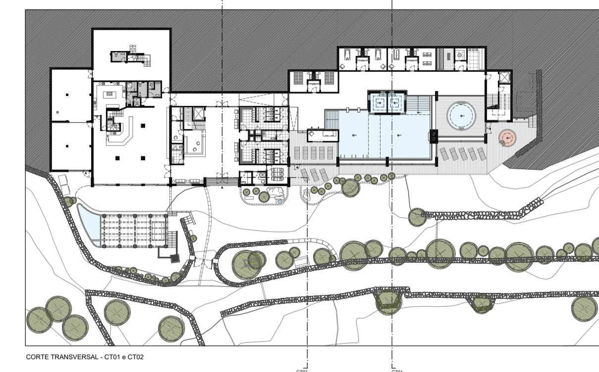
CORTE TRANSVERSAL - CT01 e CT02
