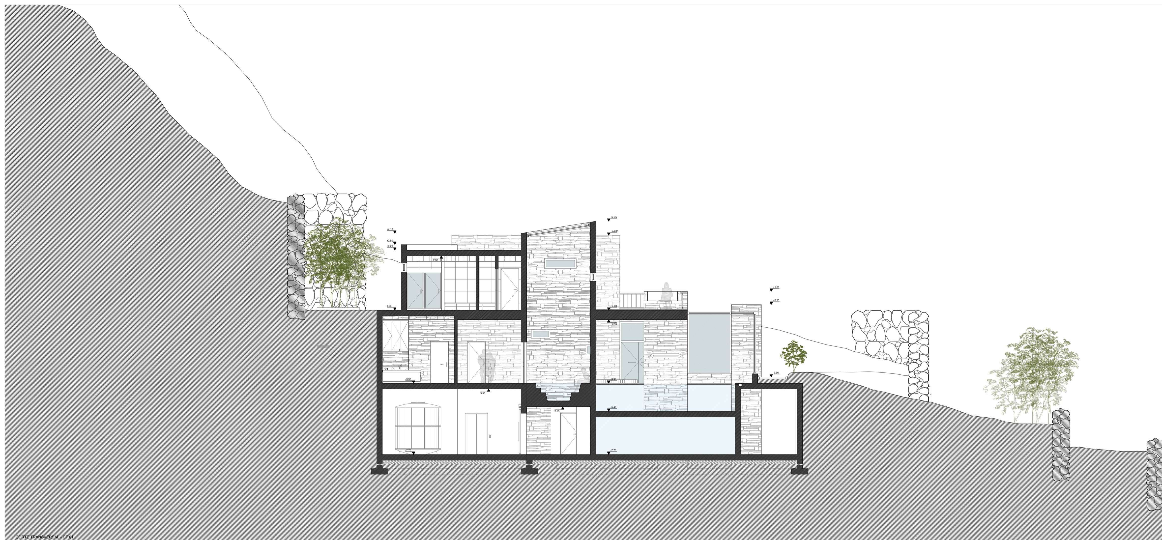
CORTE TRANSVERSAL - CT 01
