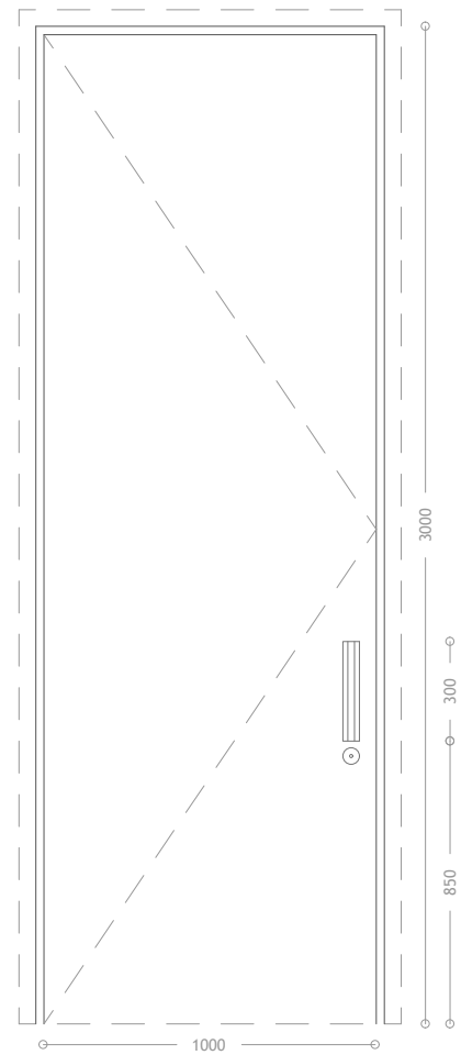
Imagem 291 - Levantamento gráfico da Porta P16 - Frente - Escala 1:25
