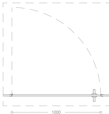
Imagem 290 - Levantamento gráfico da Porta P16 - Planta - Escala 1:25
