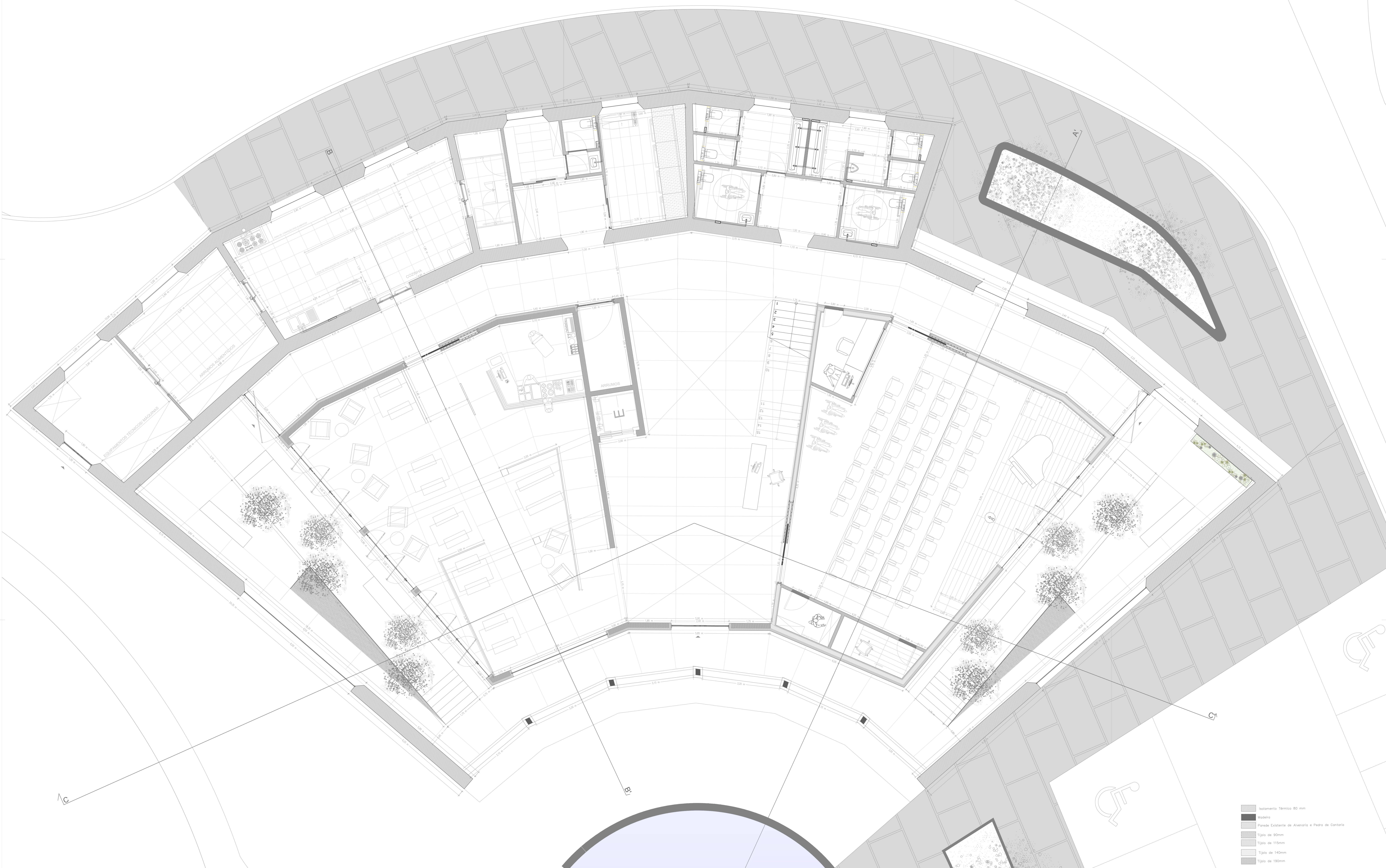
PLANTA DO PISO TÉRREO DO EDIFÍCIO DAS COCHEIRAS DOS COMBOIOS
