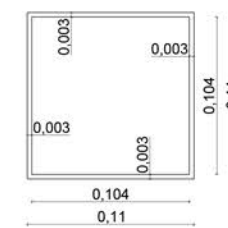
CORTE TRANSVERSAL
