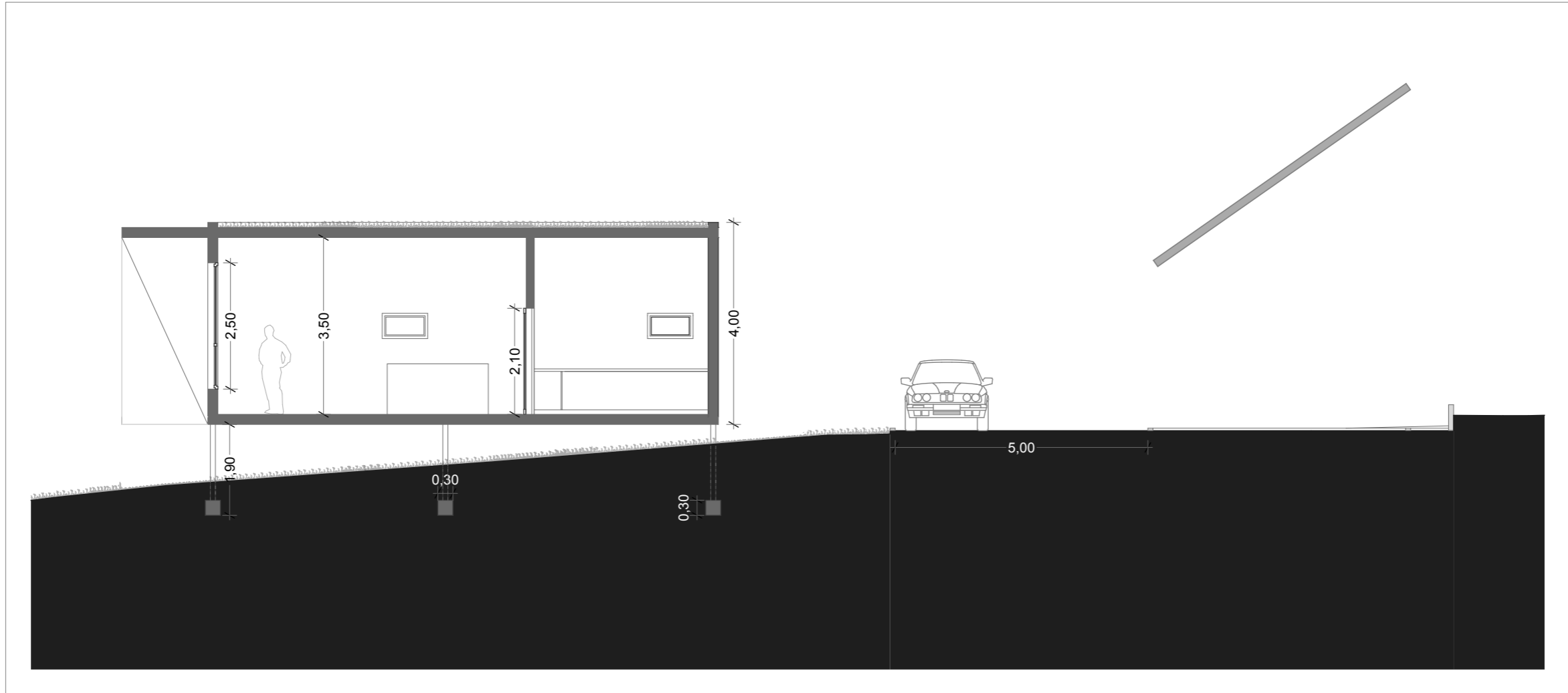
Corte A
