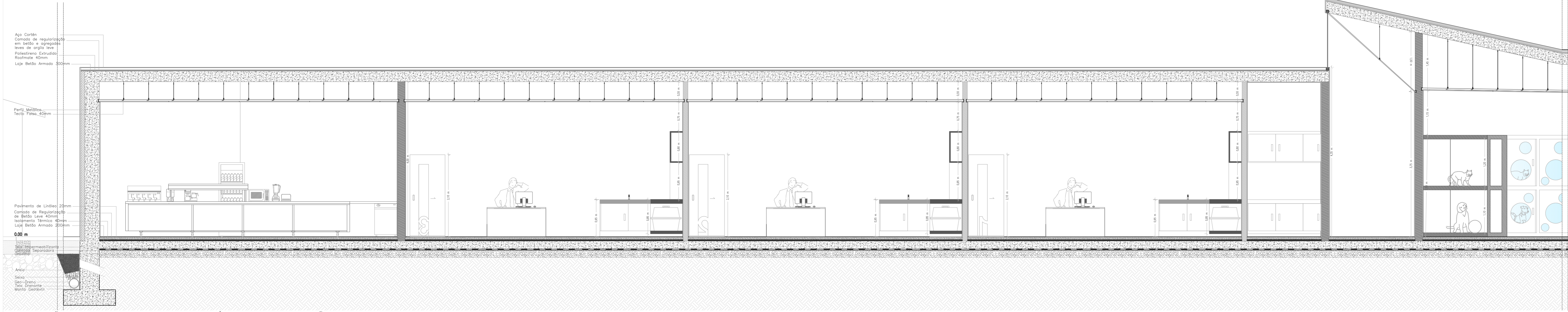
CONTINUAÇÃO DO CORTE LONGITUDINAL PELO EDIFÍCIO DA ESCOLA, RECEÇÃO E HOSPITAL
