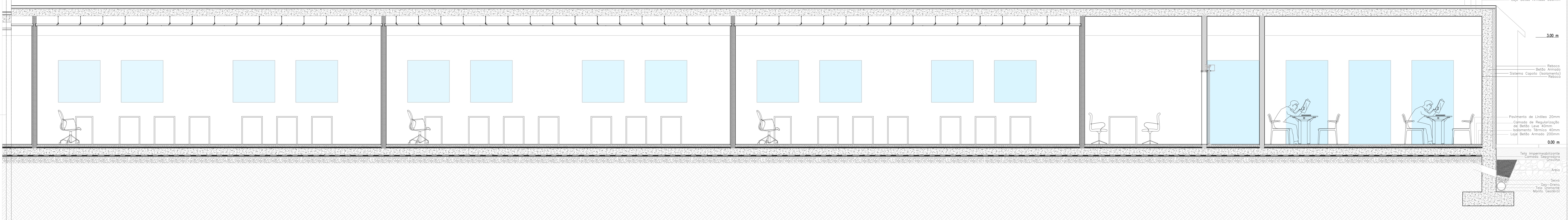
CONTINUAÇÃO DO CORTE LONGITUDINAL PELO EDIFÍCIO DA ESCOLA, RECEÇÃO E HOSPITAL
