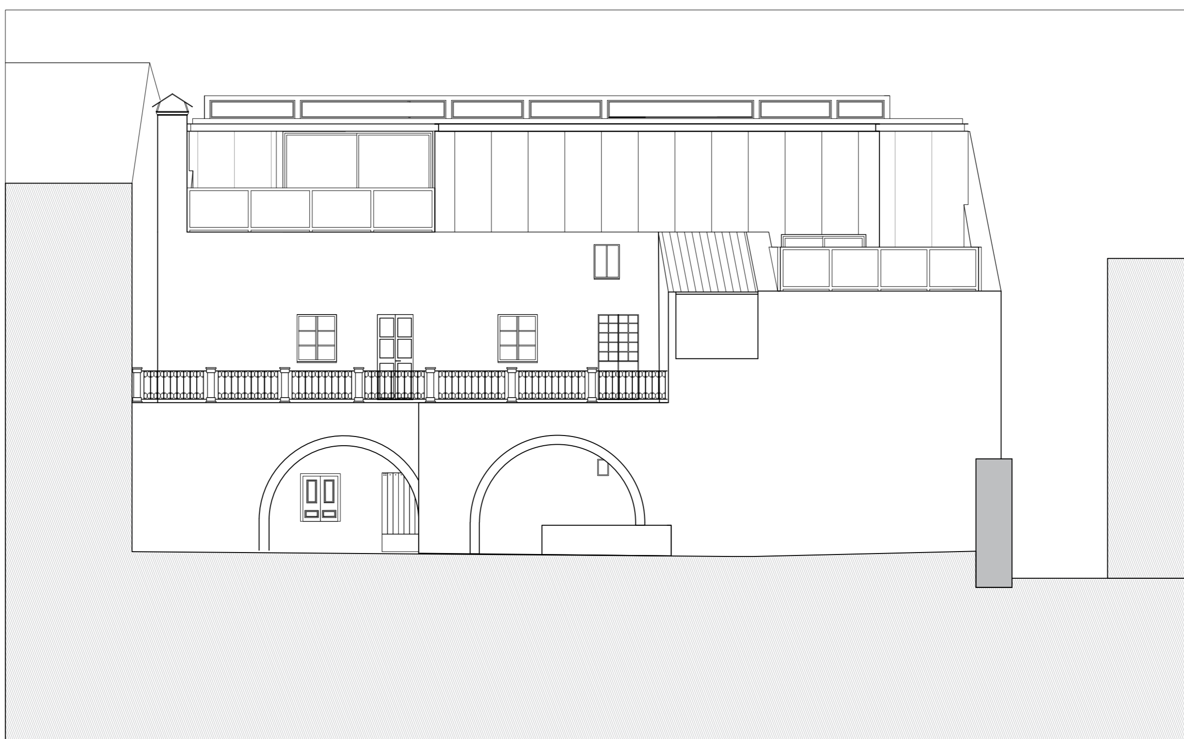
ALÇADO SUL CASA PINA FALCÃO
