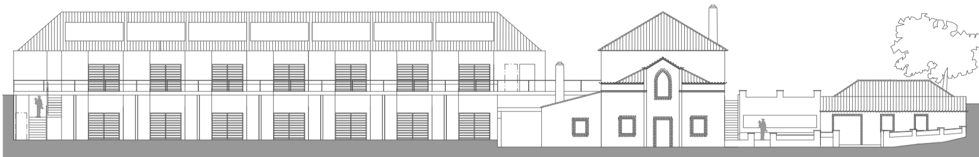
Alçado Sudoeste Escala 1:200
