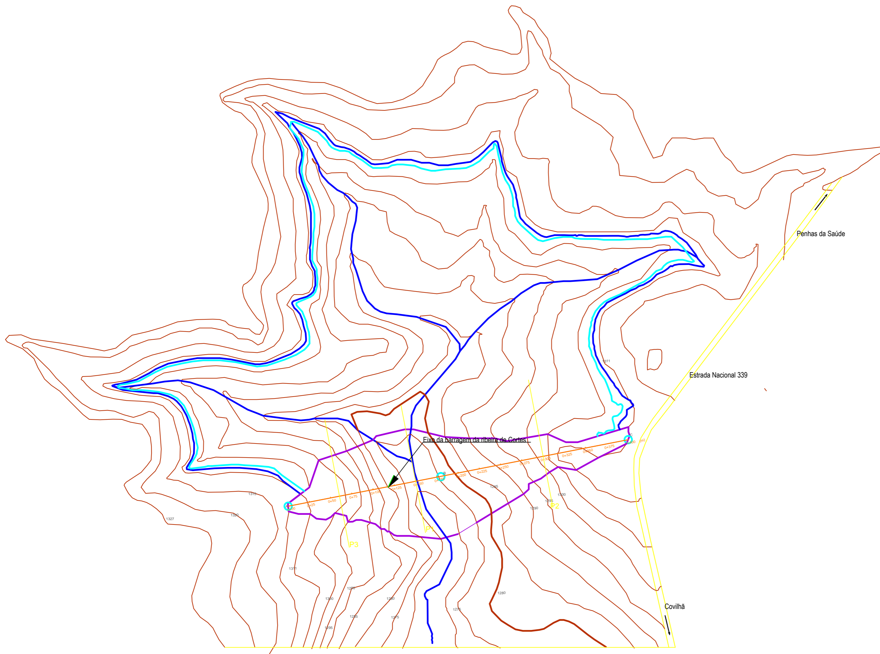
TRAÇADO DAS COTAS DO TERRENO DO EIXO DA BARRAGEM
