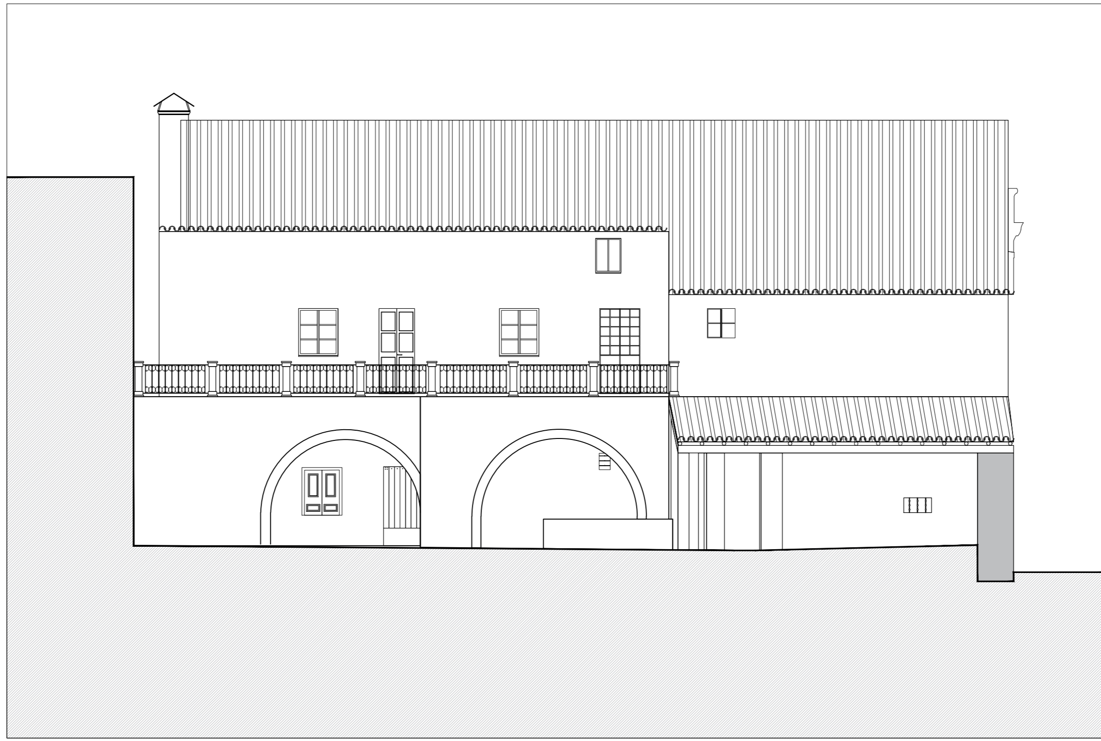
ALÇADO SUL CASA PINA FALCÃO
