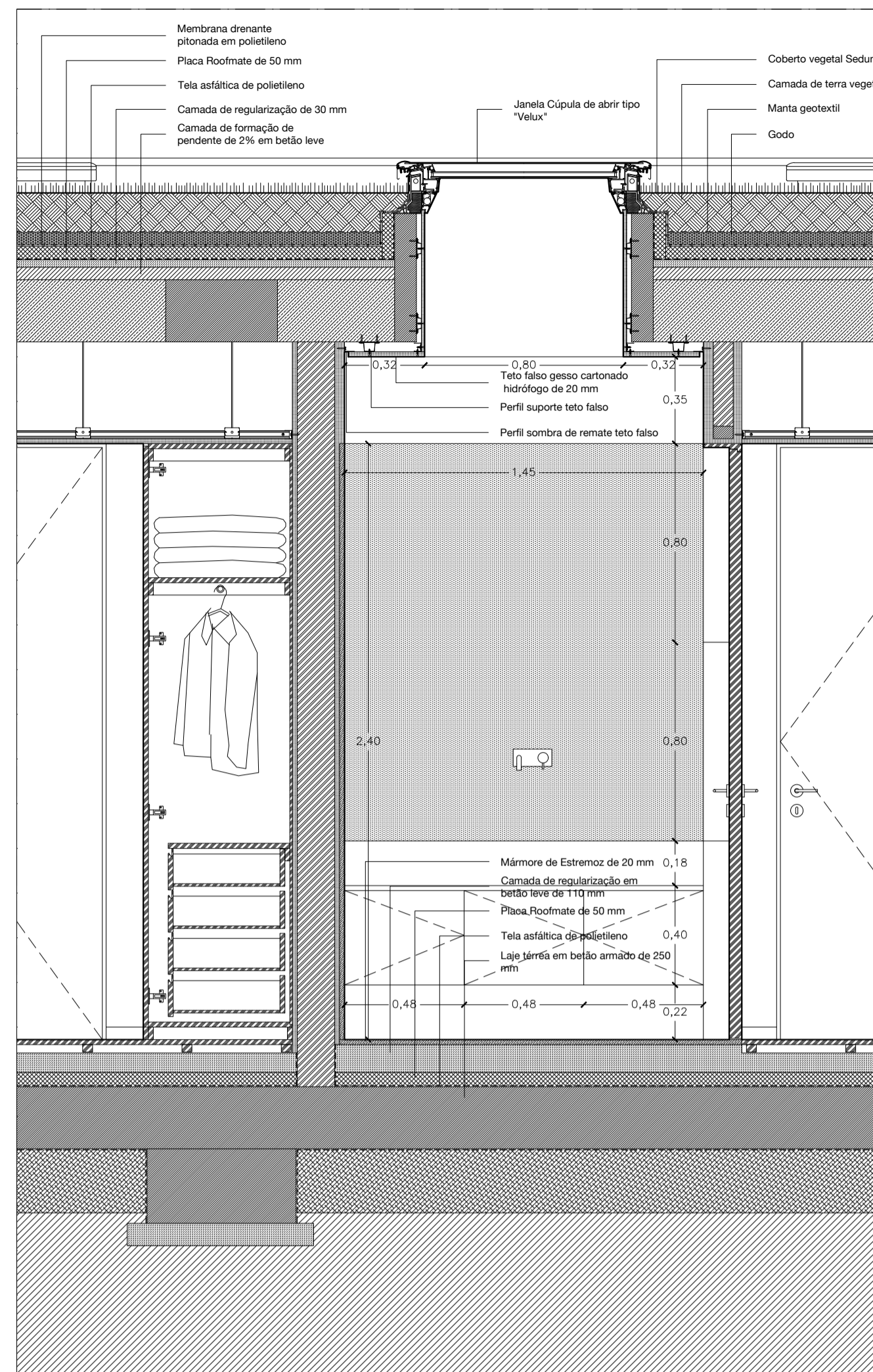
Corte a-a
