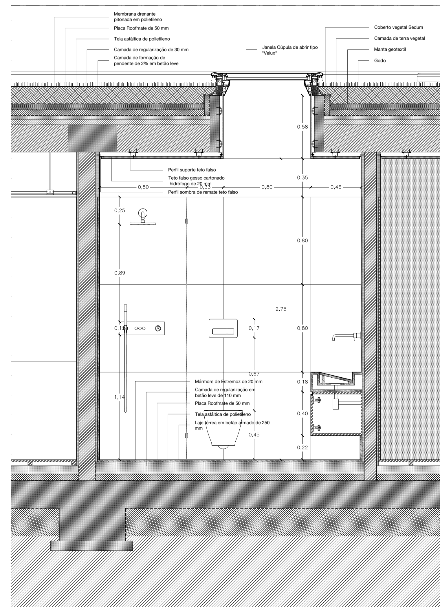
Corte d-d
