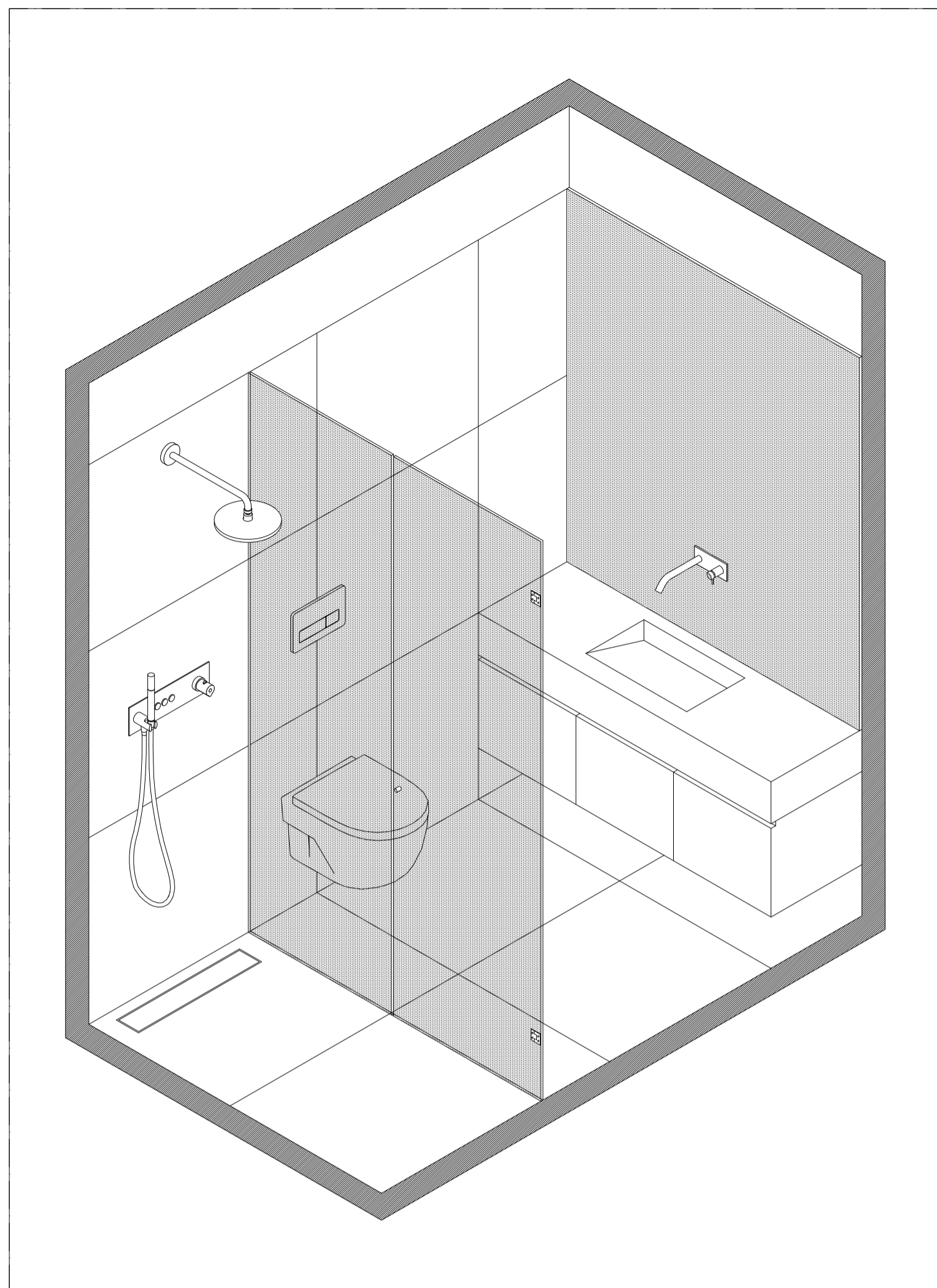
Perspectiva axonométrica
