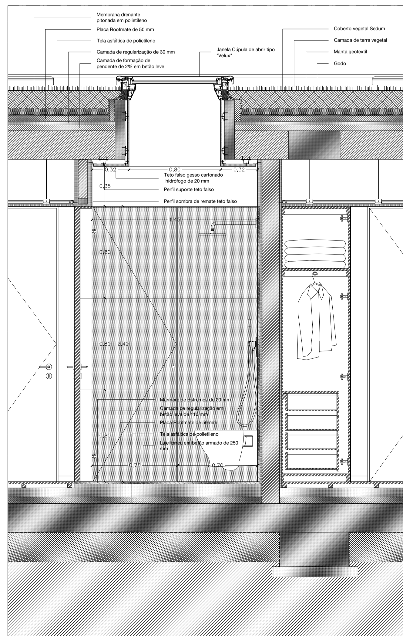
Corte c-c
