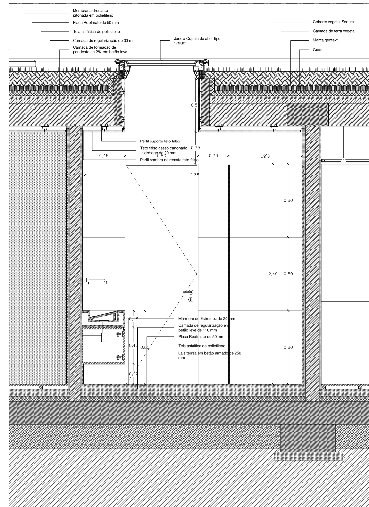
Corte b-b
