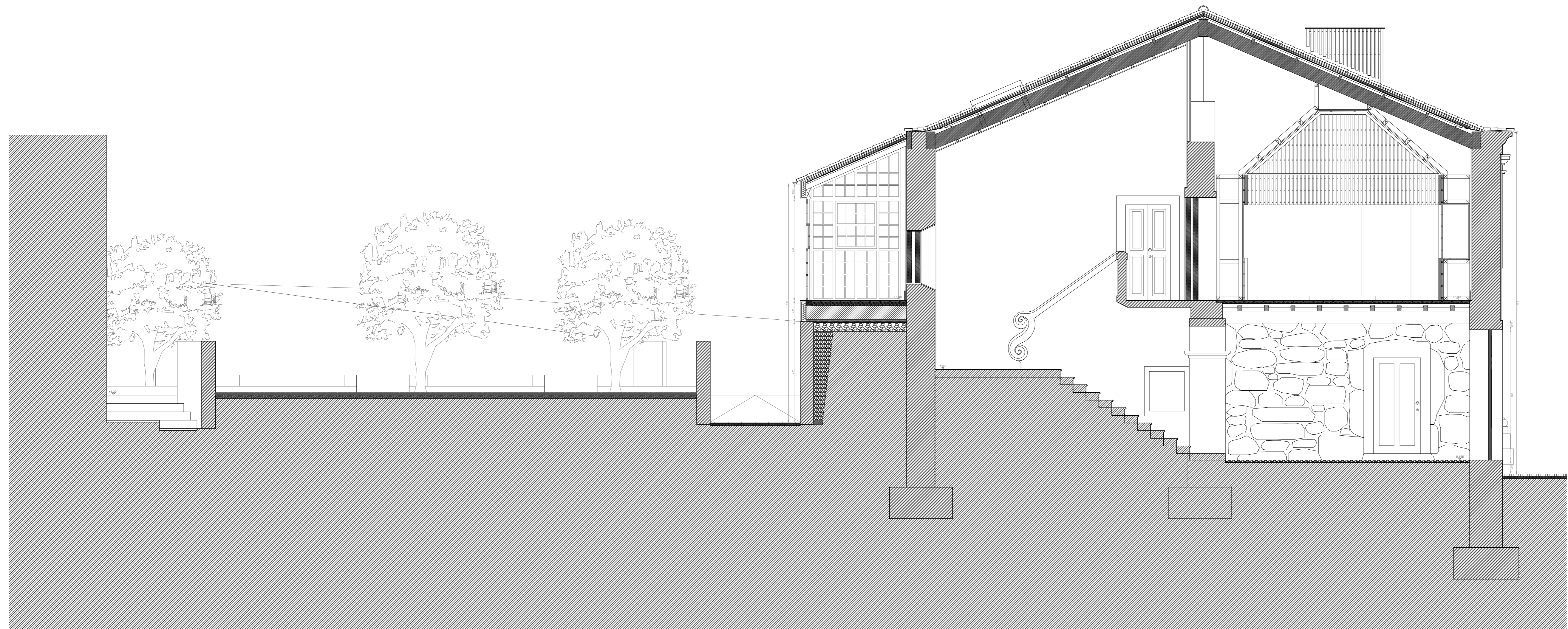
CORTE AA'
