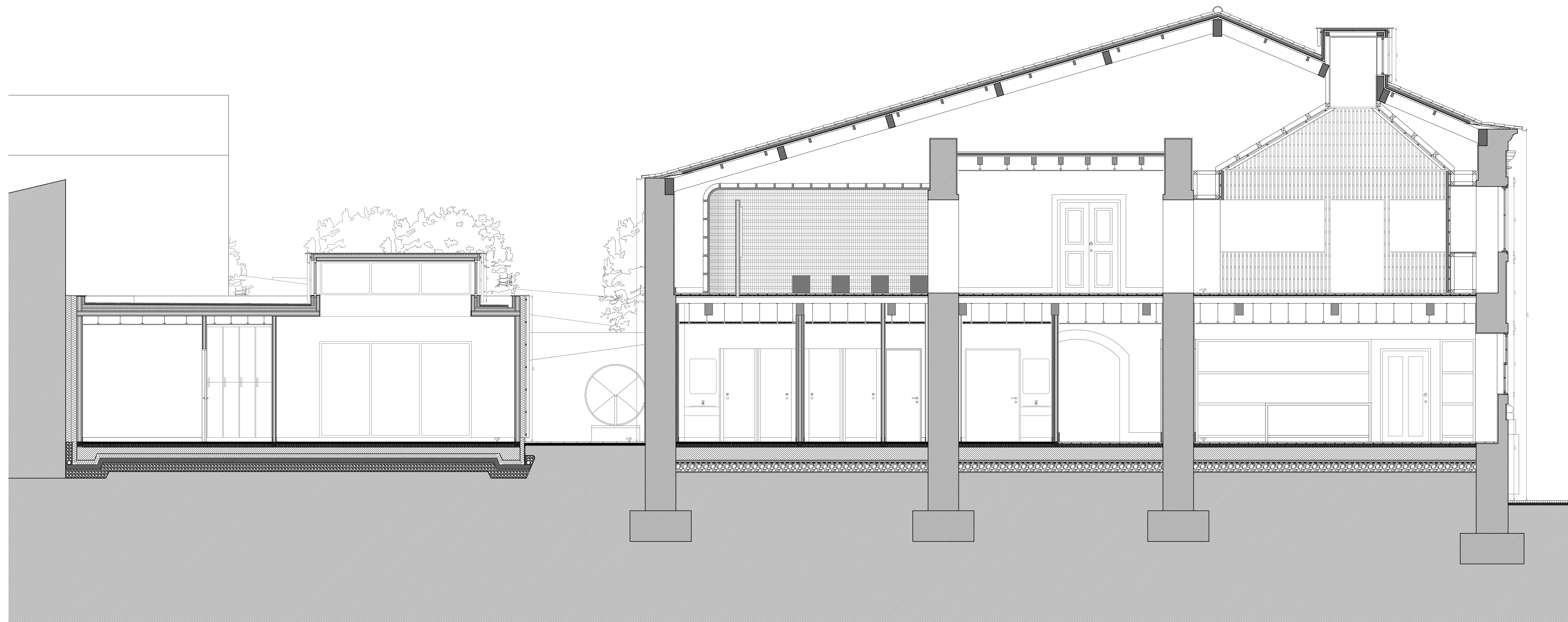
CORTE BB'
