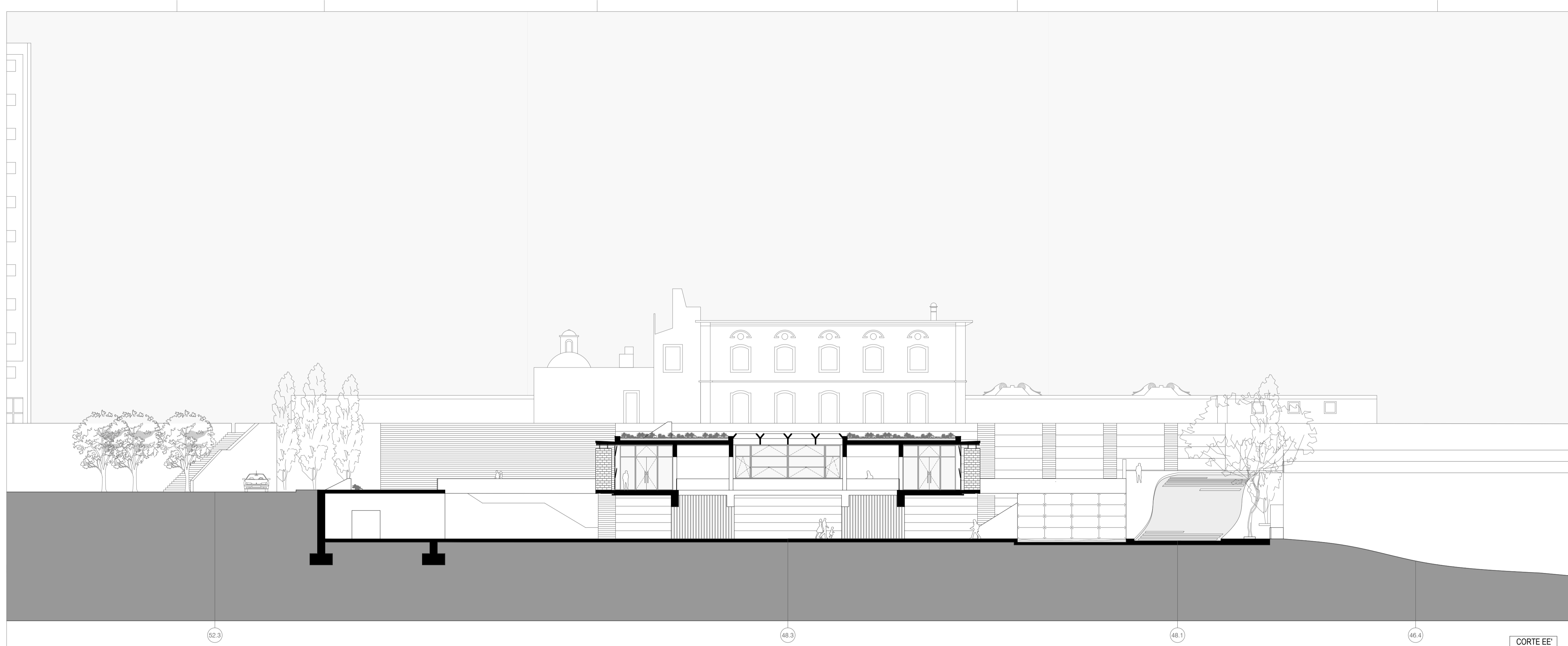
CORTE EE'
