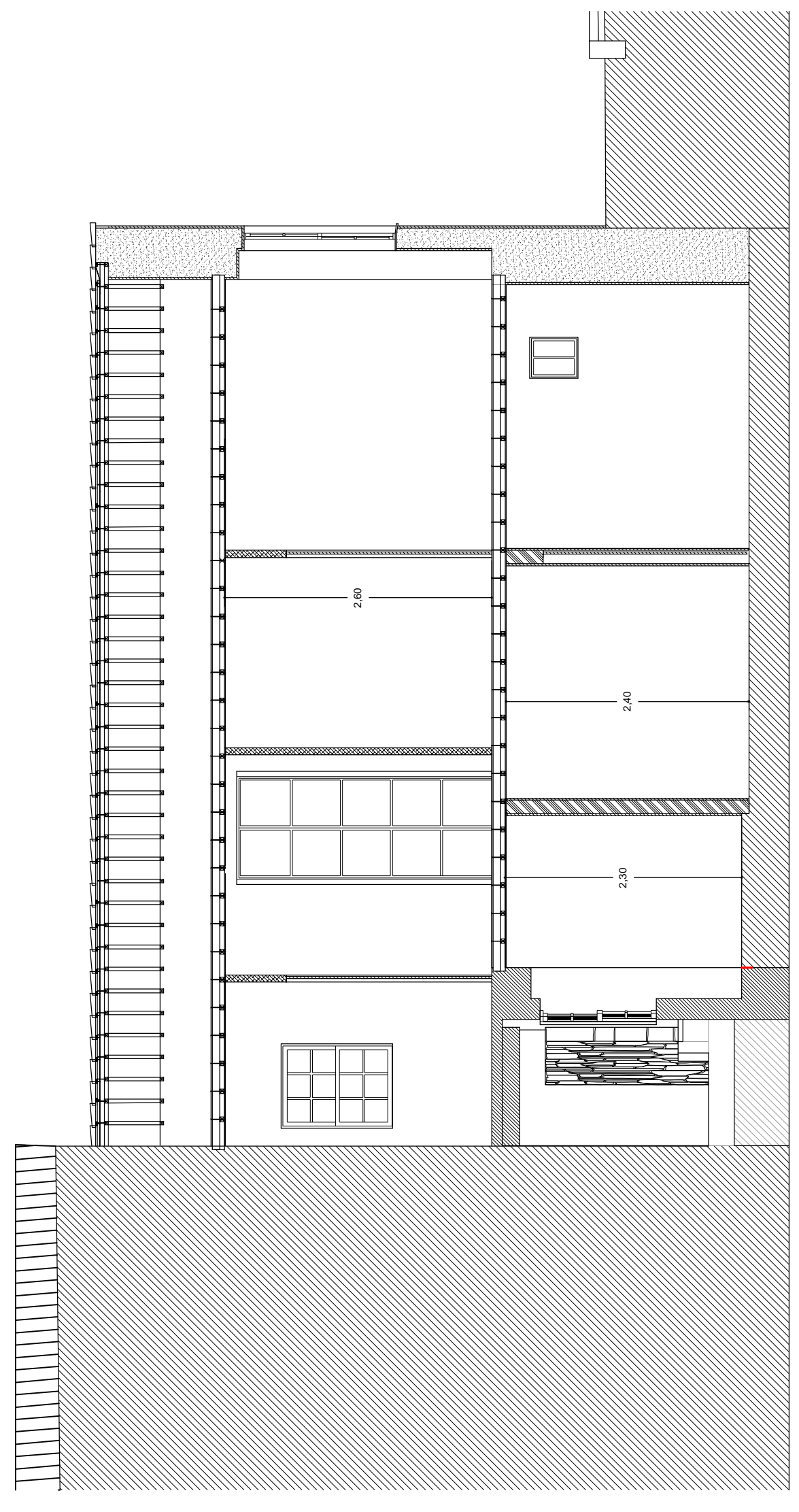
Corte A A' (Alçado Sul)
