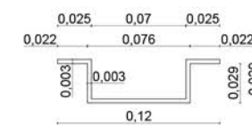
CORTE TRANSVERSAL
