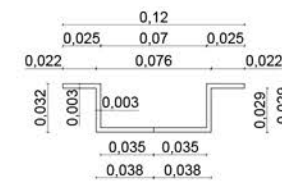
CORTE TRANSVERSAL
