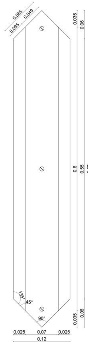
VISTA SUPERIOR
