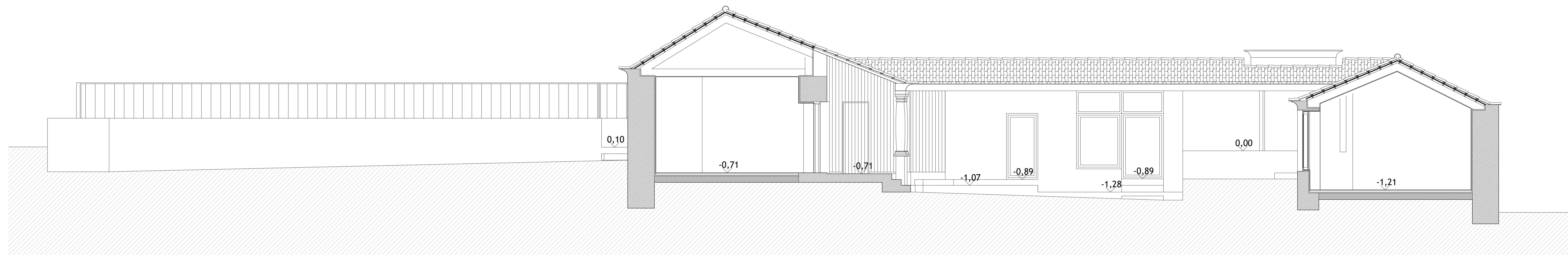
Corte CC'
