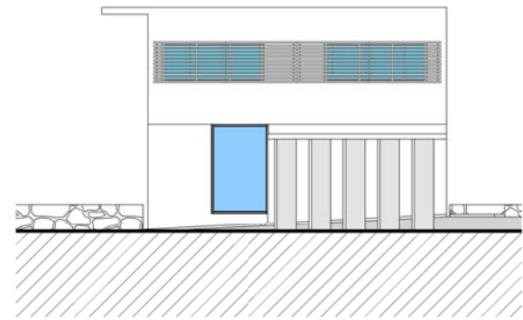
Alçado Lateral Esquerdo
