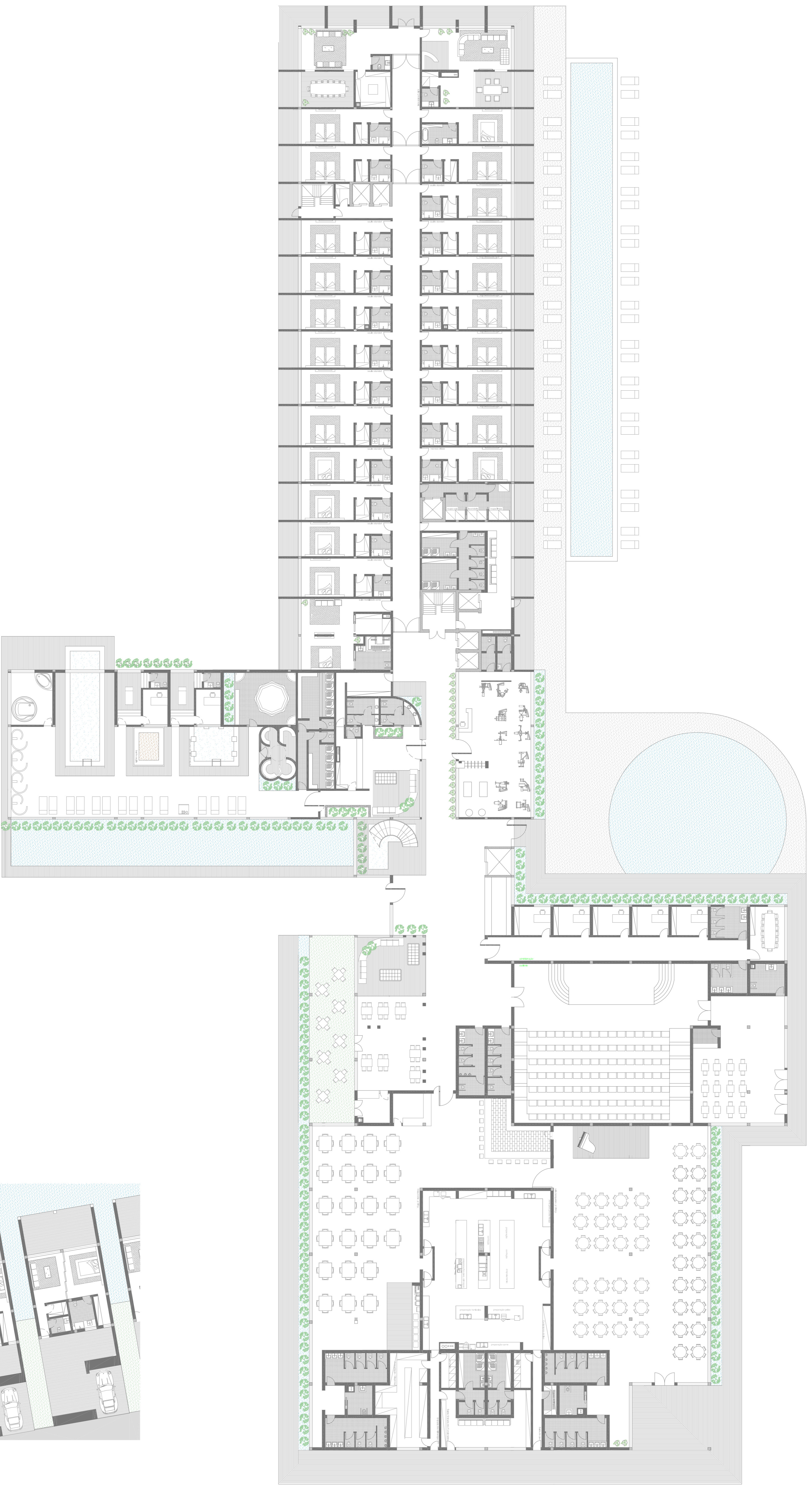
Planta tipo da habitação exterior
