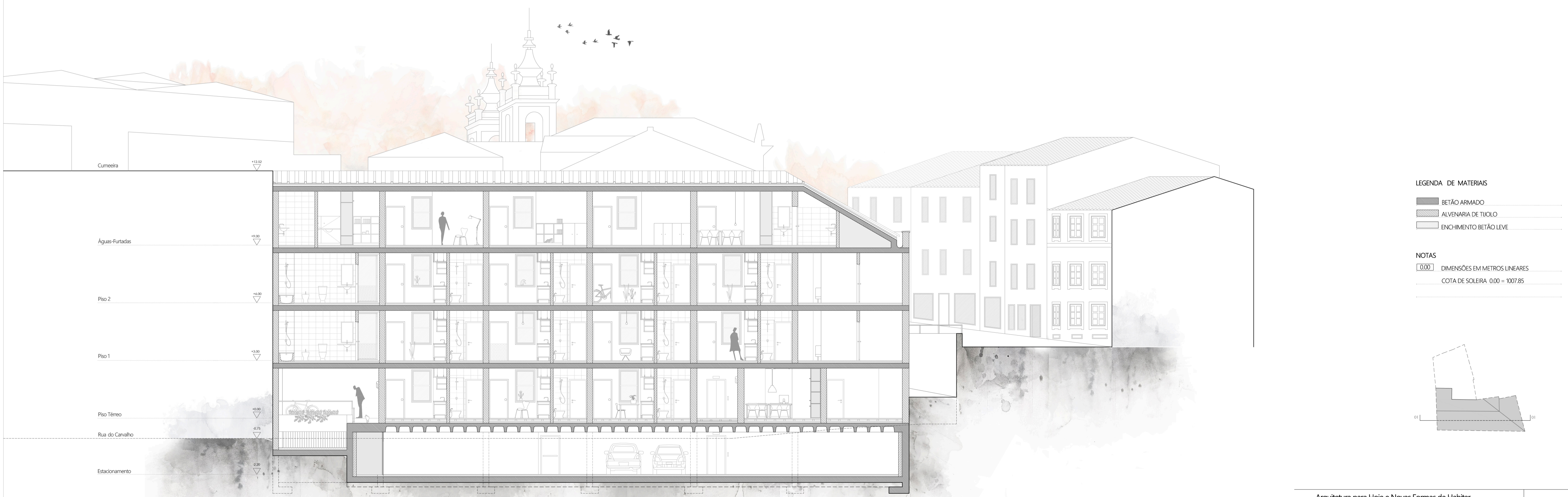
Corte Longitudinal 01
