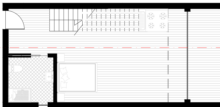
Planta Piso 1
