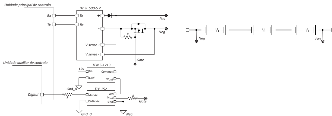
Figura 5.23: Sistema comando do circuito de potência desenvolvido.
