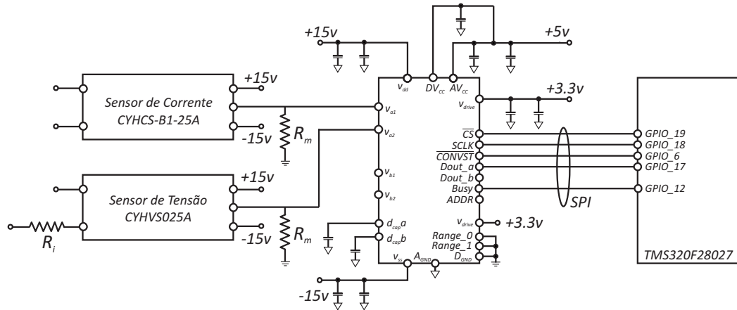
Figura 3.15: Sistema de aquisição desenvolvido.
