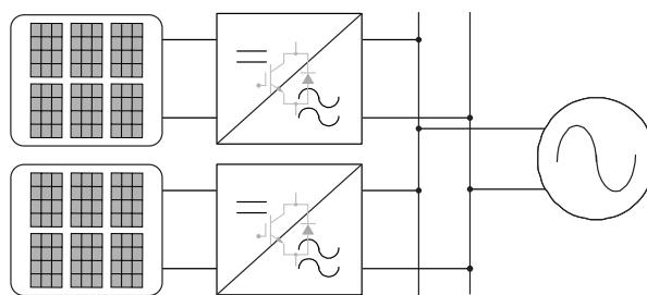
Figura 4.4: Configuração microinversora.
