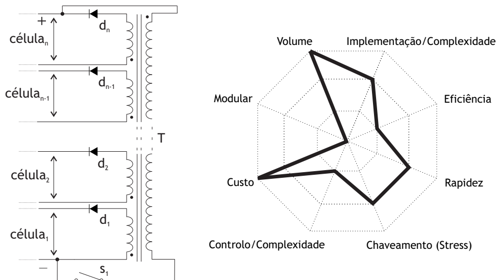
Figura 5.7: Metodologia de balanceamento multi-winding transformer : a) Circuito equivalente; b) Propriedades da metodologia.
