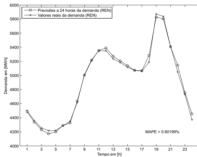
Figura 6.12: Melhor MAPE diário alcançado no dia 17-10-2015 pelo modelo de previsão da demanda (REN).
