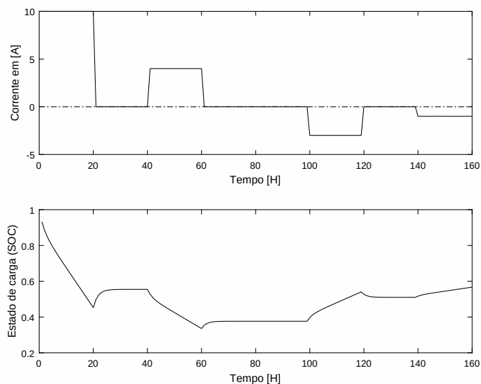
Figura F.5: Exemplo de utilização do modelo cinético de KiBaM.
