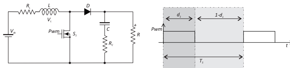
Figura C.1: Circuito elétrico e de controle do conversor boost .
