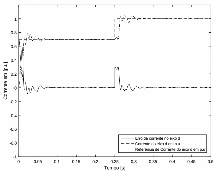
Figura 4.77: Evolução da resposta do controlador PI no eixo direto.
