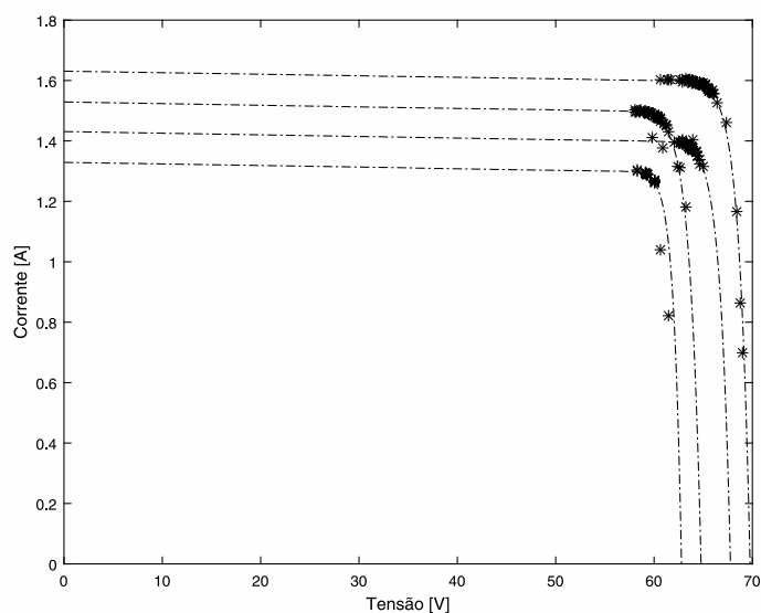
Figura 3.59: Representação gráfica dos diversos pontos de funcionamento na curva caraterística tensão-corrente.
