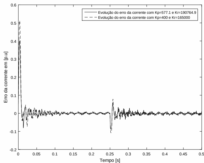
Figura 4.71: Evolução do erro da resposta do controlador PR no eixo estacionário alfa .
