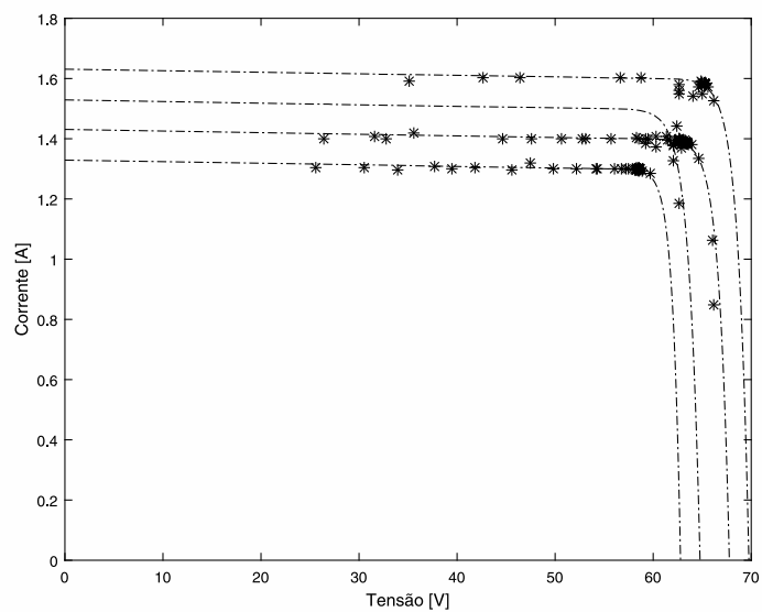
Figura 3.76: Representação gráfica dos diversos pontos de funcionamento na curva caraterística tensão-corrente.
