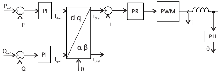
Figura 4.47: Diagrama de blocos do controlador de corrente PR.
