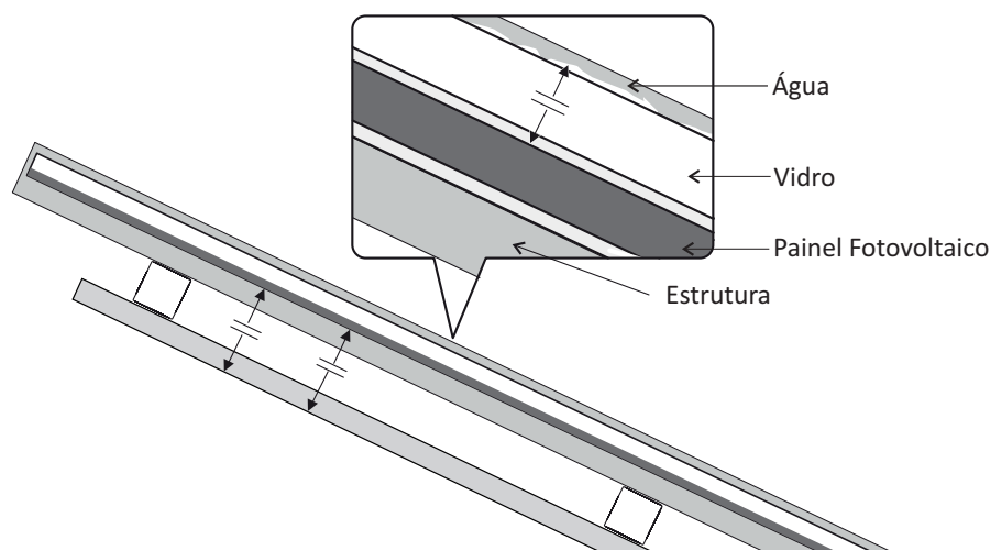
Figura 4.11: Capacidades Parasitas [54].
