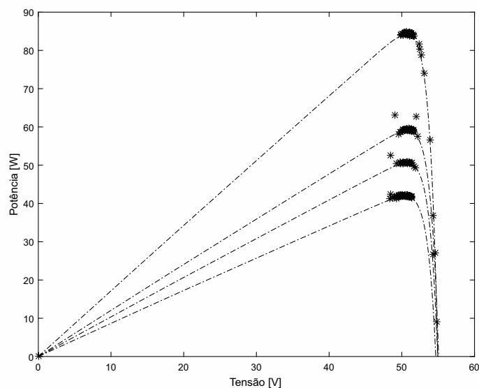
Figura 3.55: Representação gráfica dos diversos pontos de funcionamento na curva caraterística tensão-potência.
