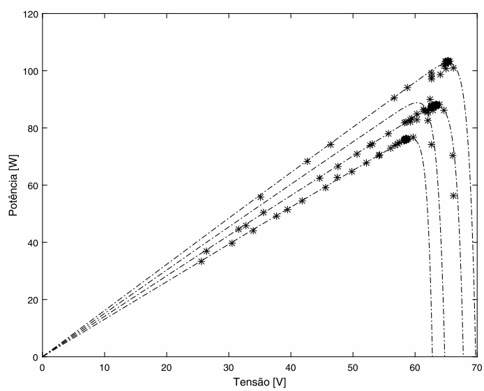
Figura 3.77: Representação gráfica dos diversos pontos de funcionamento na curva caraterística tensão-potência.
