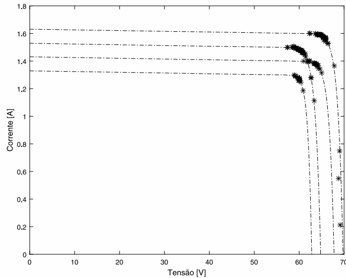
Figura 3.45: : Representação gráfica dos diversos pontos de funcionamento na curva caraterística tensão-corrente.
