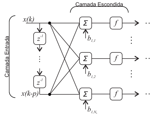
Figura B.3: Arquitetura de rede TLFNN ( Time Lagged Feedforward Neural Network ).
