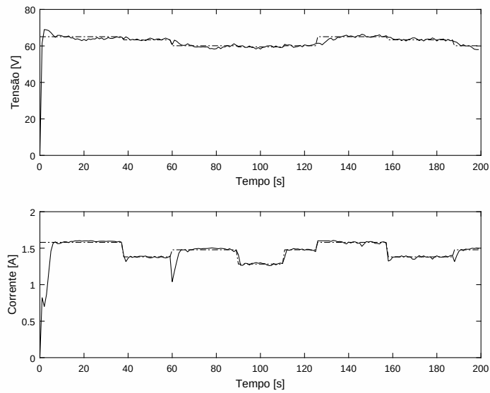
Figura 3.56: Resposta do algoritmo para o par tensão-corrente.
