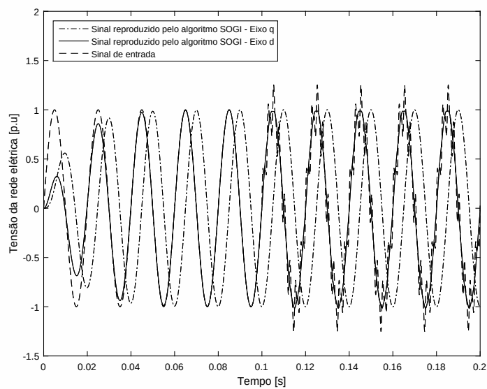
Figura 4.42: Evolução das componentes do eixo estacionário do algoritmo SOGI.
