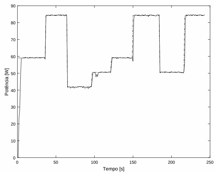
Figura 3.37: Evolução da potência.
