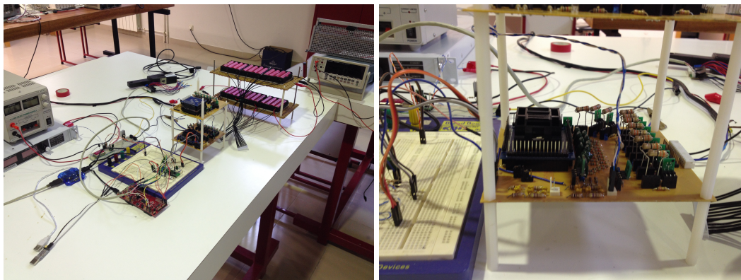
Figura 5.24: Hardware desenvolvido.
