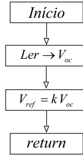
Figura 3.9: Fluxograma do algoritmo Tensão constante.
