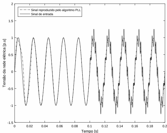
Figura 4.28: Resposta no tempo do algoritmo de sincronização PLL com filtro notch , quando submetido a várias componentes harmônicas.
