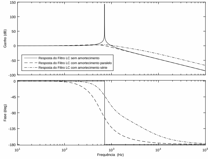
Figura 4.58: Resposta em frequência dos filtros LC com e sem amortecimento série e paralelo, com L = 5
