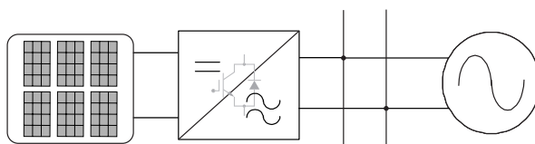
Figura 4.1: Configuração centralizada.
