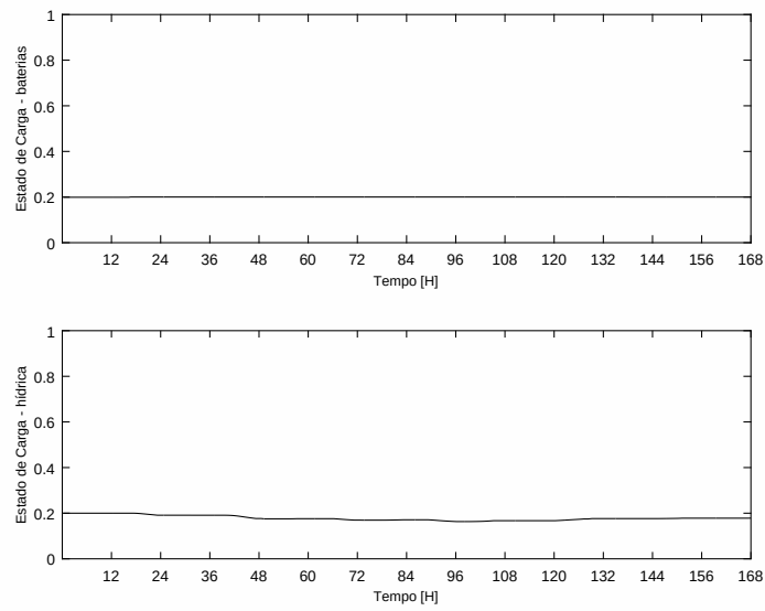
Figura 7.36: Evolução do SOC_b e SOC_h para um horizonte temporal de 168 horas.
