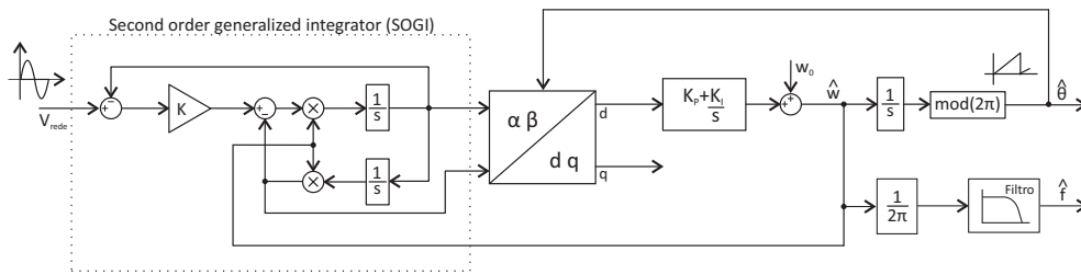
Figura 4.37: Diagrama de blocos do algoritmo de sincronização SOGI-PLL.
