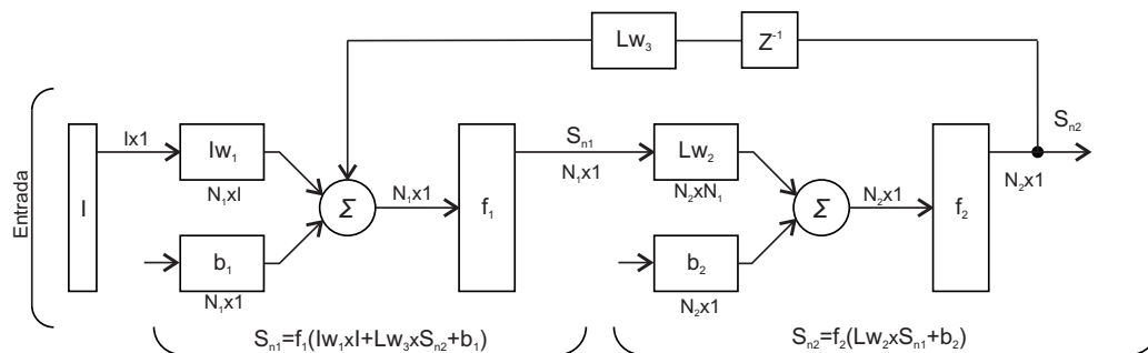
Figura B.5: Arquitetura detalhada da rede de Jordan .
