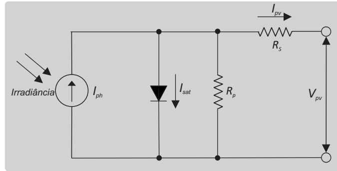
Figura 2.3: Modelo matemático a um díodo de uma célula fotovoltaica.
