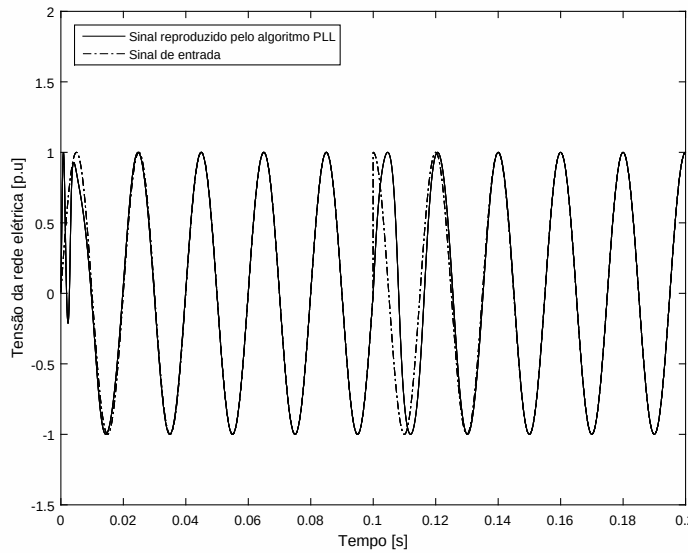
Figura 4.40: Resposta no tempo do algoritmo de sincronização SOGI-PLL, quando submetido a um salto de fase de \frac{\pi}{2} .
