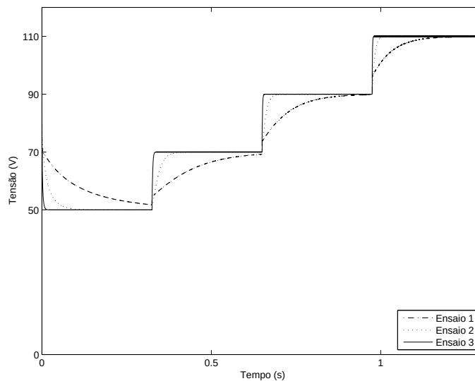
Figura 3.20: Resposta do sistema para diferentes tensões de referência.
