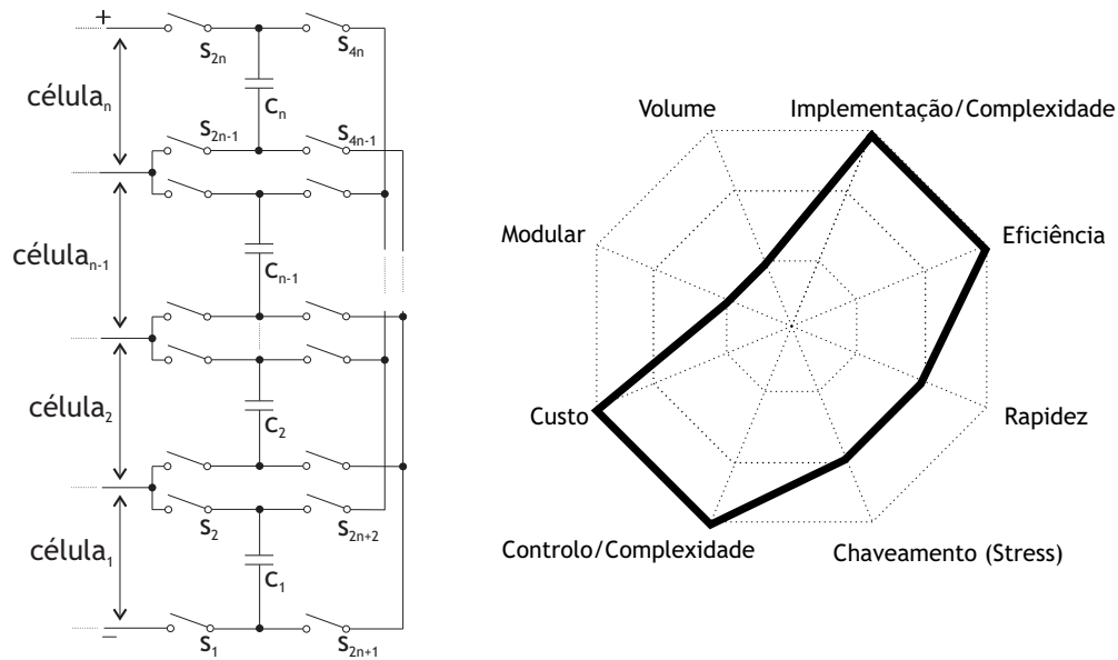
Figura 5.6: Metodologia de balanceamento series-parallel switched capacitor : a) Circuito equivalente; b) Propriedades da metodologia.
