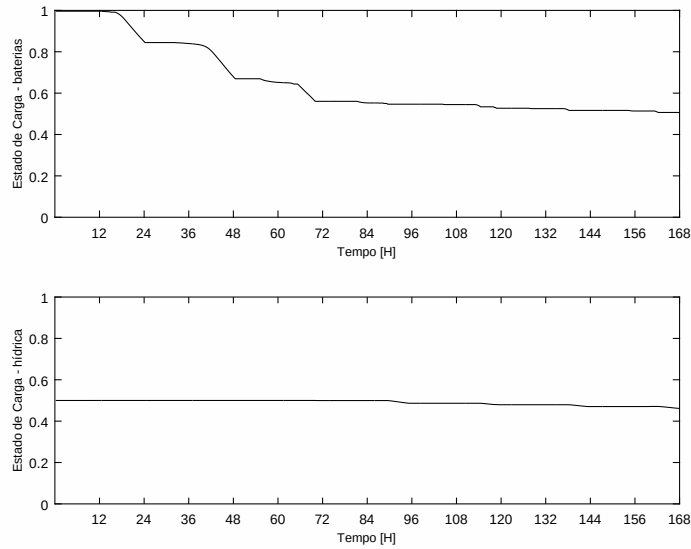
Figura 7.26: Evolução do SOC_b e SOC_h obtido para um horizonte temporal de 168 horas.
