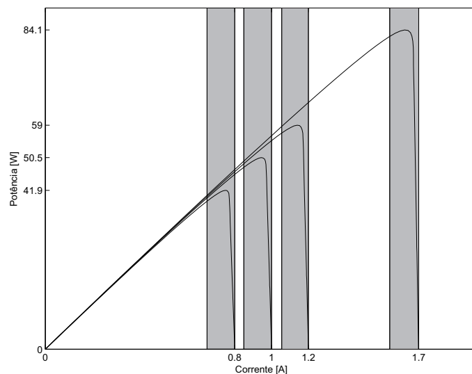
Figura 3.33: Variação da corrente em torno do ponto de máxima potência.
