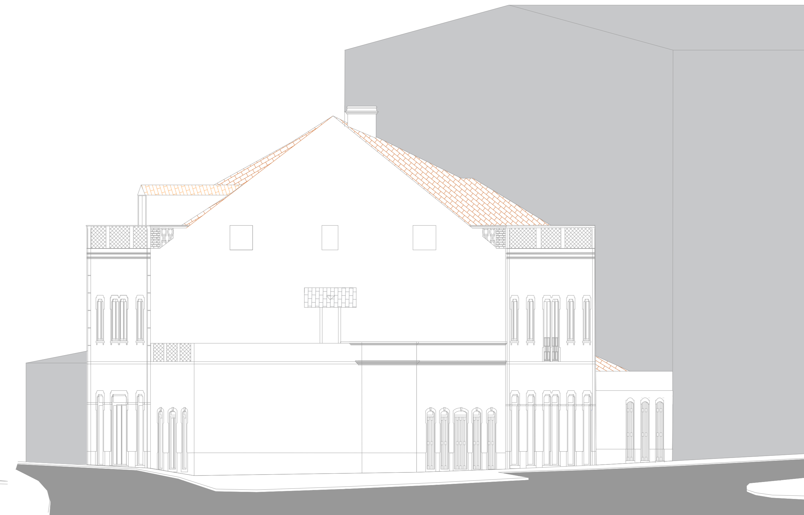
Alçado Sul
