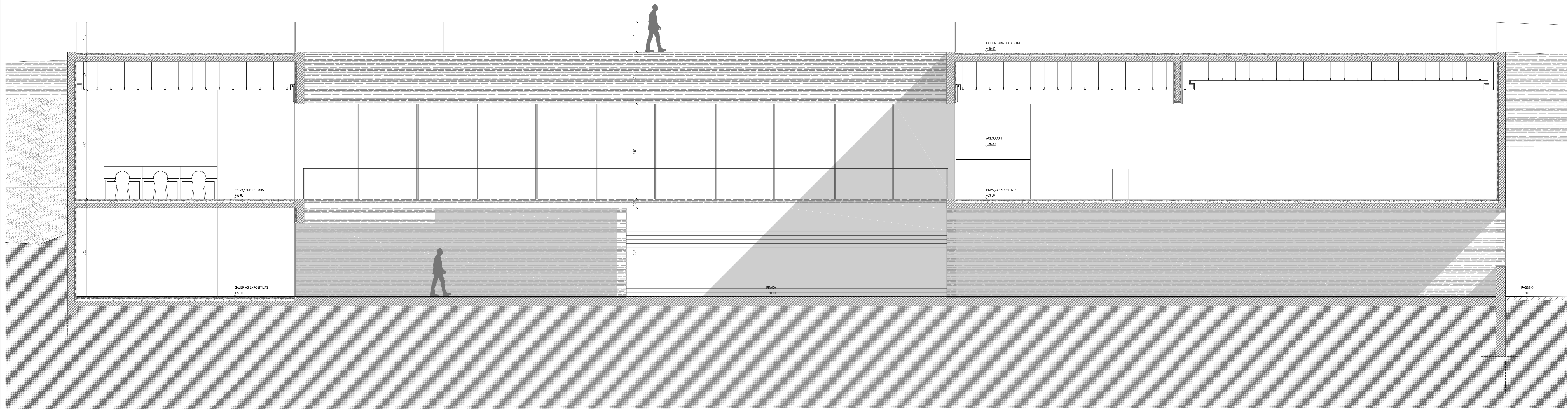
CORTE TRANSVERSAL 2
