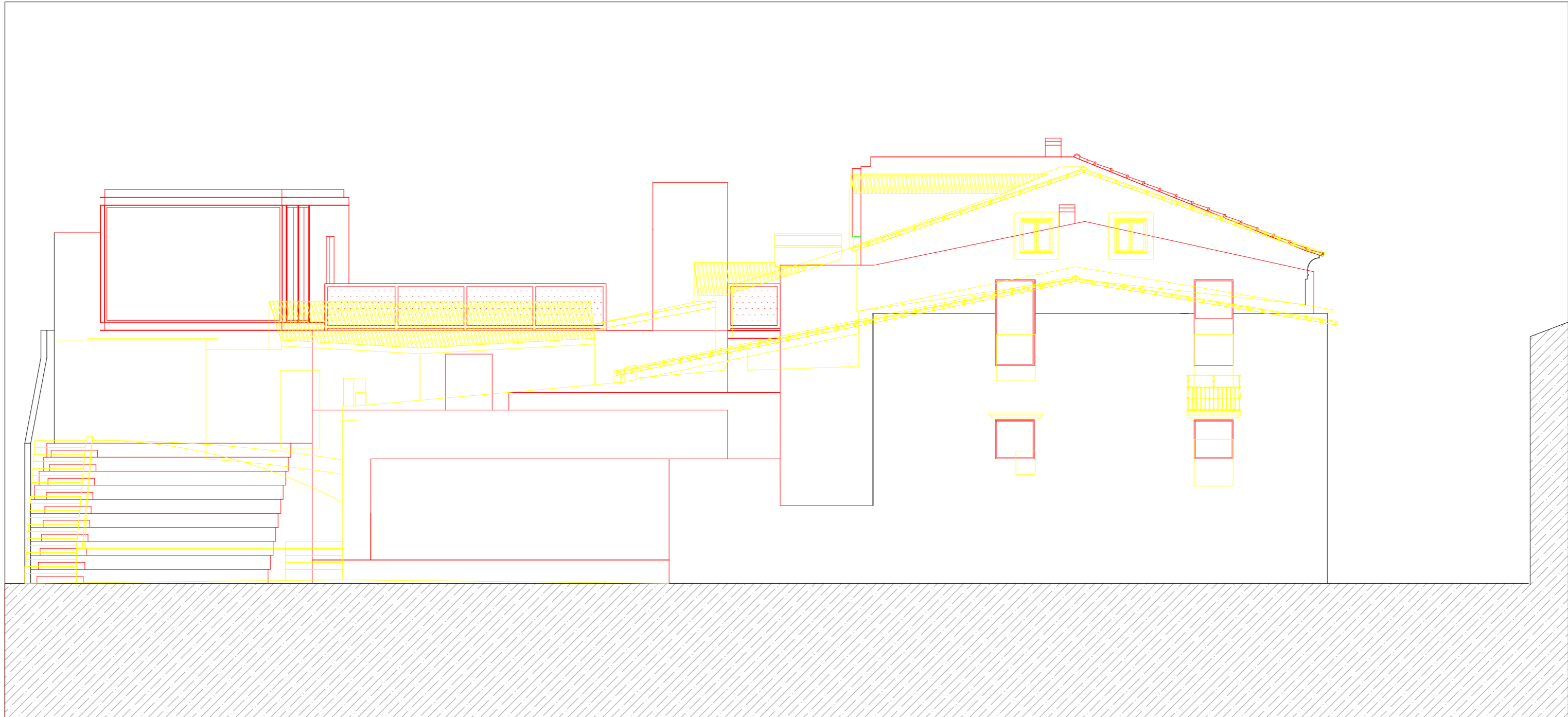
ALAÇADO SUL ANEXO CASA PINA FALCÃO V.A
