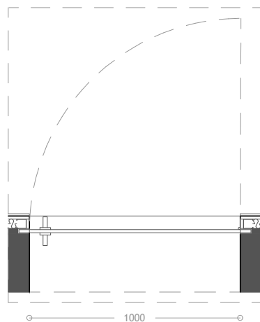
Imagem 294 - Levantamento gráfico da Porta P17 - Planta - Escala 1:25
