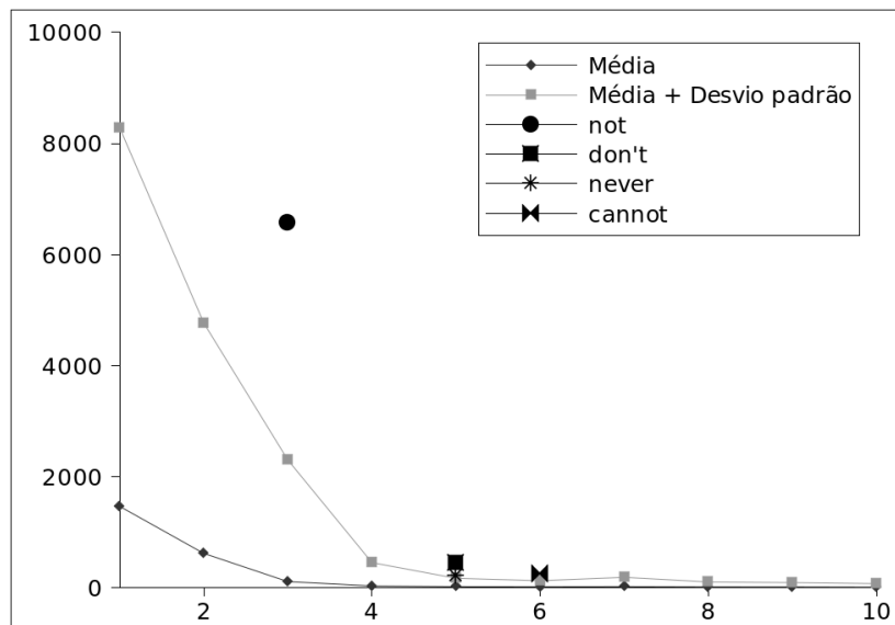
Figura 3.2: Gráfico da frequência média das palavras em inglês
