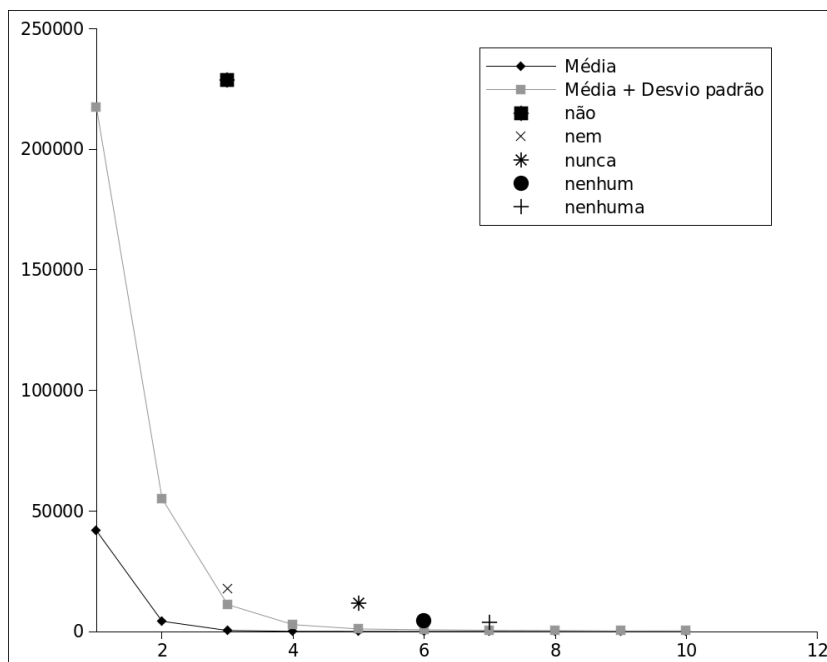
Figura 3.1: Gráfico da frequência média das palavras em português
